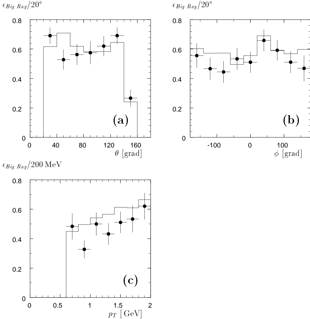
Abbildung 5.6: Die Ansprechwahrscheinlichkeit für Big-Ray-Signale in Abhängigkeit vom Winkelbereich (a), (b) nach dem Durchgang einer Spur durch das zugehörige räumliche Proportionalkammersegment. Abbildung (c) zeigt das Ansprechverhalten der Proportionalkammersegmente in Abhängigkeit vom Transversalimpuls der Spur. Für die Daten (Punkte) und die Monte-Carlo-Ereignisse wurde die Selektion nach Tabelle 5.3 durchgeführt. Die Monte-Carlo-Simulation ist als Histogramm überlagert dargestellt.
