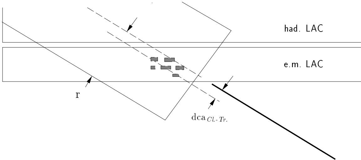
Abbildung 4.5: Die Skizze zeigt die Interpolation der rekonstruierten Spur vom Spurkammersystem zum LAC.
