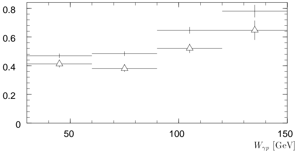
Abbildung 5.9: Die gesamte Triggerakzeptanz für L1 und L4 in Abhängigkeit von der \gamma p -Schwerpunktsenergie. Die Akzeptanzen wurden anhand des Monte-Carlo-Modells für protonelastische Ereignisse (Balken) und für Ereignisse mit Protondissoziation (Dreiecke) ermittelt.
