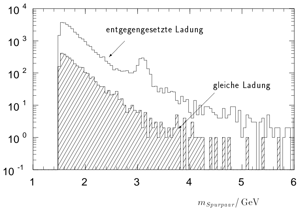
Abbildung 4.3: Die Abbildung zeigt die Massenverteilung für die selektierten Zwei-spurereignisse. Ereignisse mit einer Myonspur im instrumentierten Eisen wurden unterdrückt. Deutlich ist das J/\psi -Signal für die entgegengesetzt geladene Spurkombination erkennbar. Der Anteil an Ereignissen mit gleich geladener Spurkombination beträgt etwa 10 %. Es wurden Spuren in einem Polarwinkelbereich 20^\circ < \theta < 160^\circ zugelassen.
