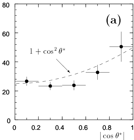
Abbildung 6.5: Abbildung (a): Auf Detektoreinflüsse korrigierte Zerfallswinkelverteilung im Vergleich zur Vorhersage transversal polarisierter J/\psi -Mesonen (Gleichung: 6.6). (b) zeigt für J/\psi -Mesonen die Polarakzeptanz nach dem Polarwinkelschnitt auf die beiden Zerfallsleptonen von 20^\circ < \theta < 160^\circ sowie die Detektorakzeptanz, die innerhalb des Polarwinkelbereichs ermittelt wurde.
