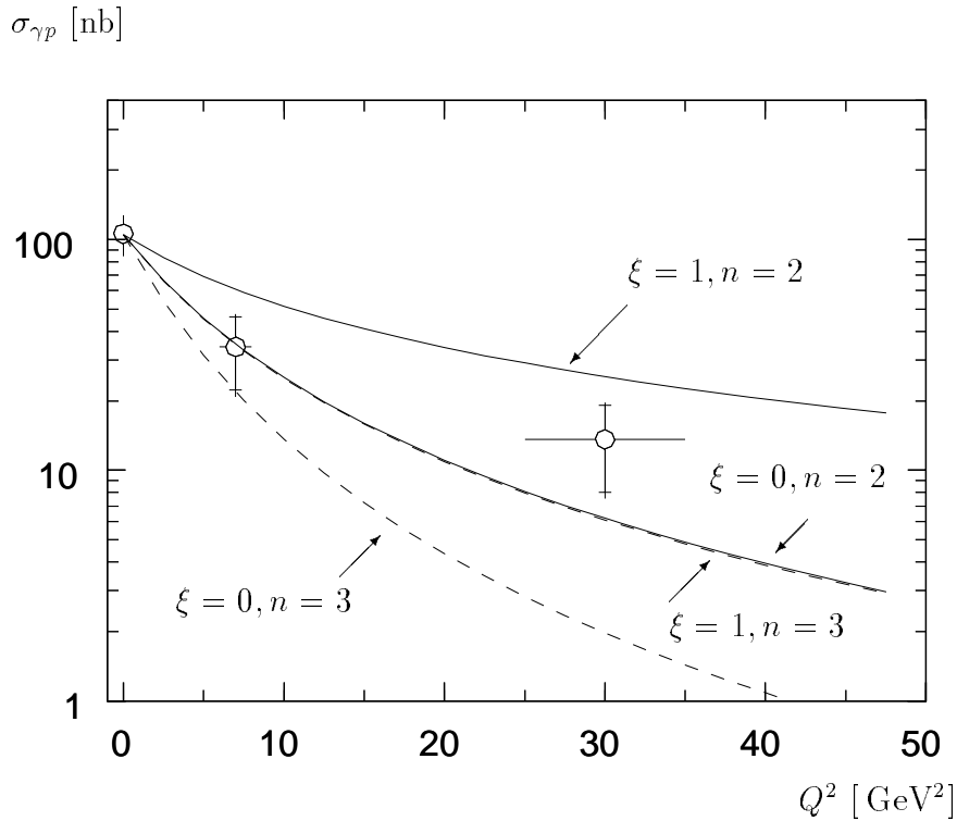
Abbildung 6.7: Der \gamma p -Wirkungsquerschnitt in Abhängigkeit von Q^2 . Das Abfallen von \sigma_{\gamma p}(Q^2) wird in zwei verschiedene Bereiche je nach dem Potenzverhalten n unterteilt. Die durchgezogene Kurve steht für n = 2 und der gestrichelte Kurvenverlauf für n = 3 . \xi = 1 bildet die obere und \xi = 0 die untere Grenze ( n, \xi beziehen sich auf Glg. 6.8).
