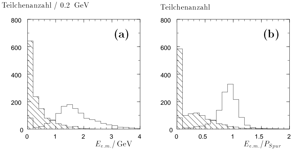
Abbildung 4.6: Vergleich zwischen Elektronen aus dem Zerfall des J/\psi -Mesons (Monte-Carlo-Modell) und Pionen aus Photoproduktionsdaten. Abbildung (a) zeigt die Energieverteilung der Elektronen und Pionen nach der Rekonstruktion der elektromagnetischen Energie im LAC und Abbildung (b) das Verhältnis zwischen rekonstruierter Energie im LAC und dem Impuls des Spurkammersystems. Elektron- und Pionverteilungen (schraffiert) sind auf die gleiche Anzahl von Einträgen normiert.
