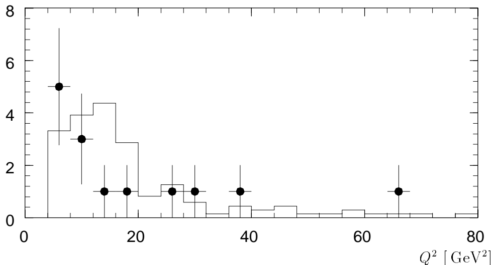
Abbildung 6.6: Q^2 -Verteilung der J/\psi \rightarrow e^+e^- DIS-Kandidaten. Die Monte-Carlo-Vorhersage des VMD-Modells ist als Histogramm überlagert dargestellt.
