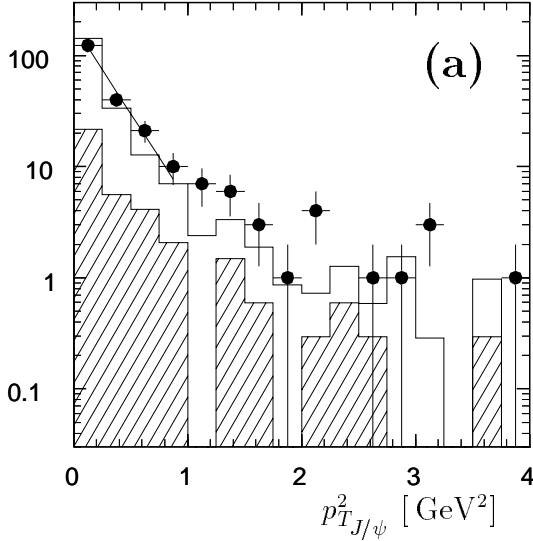
Abbildung 6.3: Abbildung (a) zeigt p_{T,J/\psi}^2 für die Vorwärtsselektion V . Wie in Abbildung 6.2 werden hier Daten und Monte-Carlo-Modell überlagert. Das Histogramm zeigt die Summe aus protonelastischen und inelastischen Ereignissen. Der protoninelastische Anteil ist schraffiert dargestellt. Abbildung (b) zeigt dieselbe Verteilung nach der Selektion NV .
