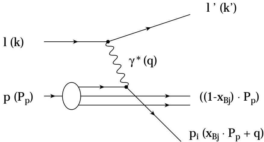
Abbildung 1.1: Tiefinelastische Elektron–Proton–Streuung. Das einlaufende Lepton trägt die Bezeichnung l mit dem Viererimpuls (k) . Für die weiteren Teilchen ist analog dazu der Teilchentyp und Viererimpuls definiert.
