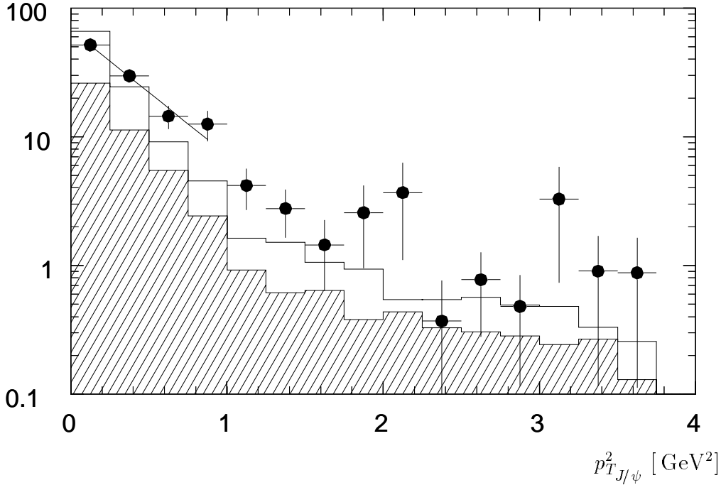
Abbildung 6.2: Die Transversalimpulsverteilung des rekonstruierten J/\psi -Mesons im Vergleich zwischen Daten und Monte-Carlo-Modell für J/\psi -Kandidaten mit Q^2 < 4 \text{ GeV}^2 . Die Punkte repräsentieren Daten und das Histogramm das Monte-Carlo. Der Monte-Carlo-Anteil mit Protondissoziation ist schraffiert gekennzeichnet.
