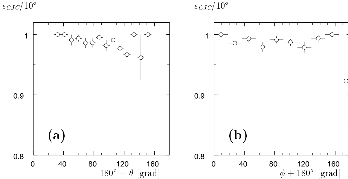
Abbildung 5.1: Nachweiswahrscheinlichkeit einer Spur im CJC-Spurkammersystem ermittelt durch kosmische Myonen: Abbildung (a) zeigt die Abhängigkeit vom Polarwinkel. (b) zeigt den Azimutalbereich.
