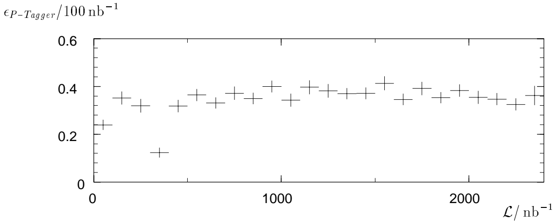
Abbildung 5.11: Relative Trefferhäufigkeit der Zählkanäle 0,1,3,5 des Proton-Taggers in Abhängigkeit von der Luminosität für das Ansprechen von mindestens einem Kanal.
