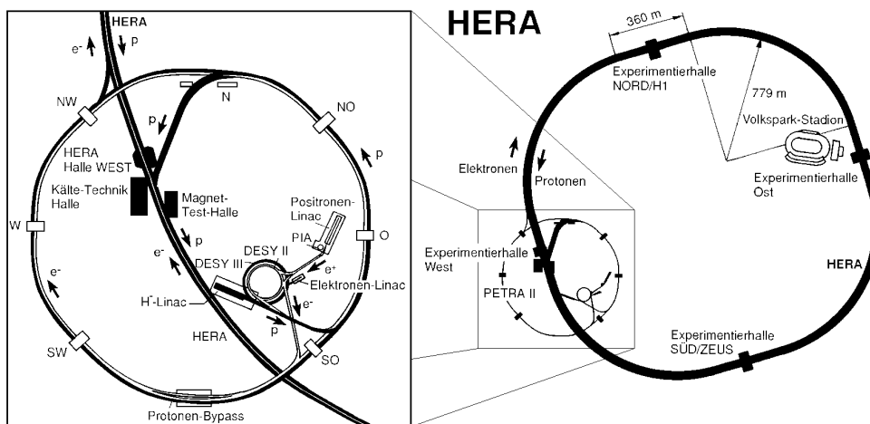
Abbildung 2.1: Die Speicherringanlage HERA und ihre Vorbeschleuniger
