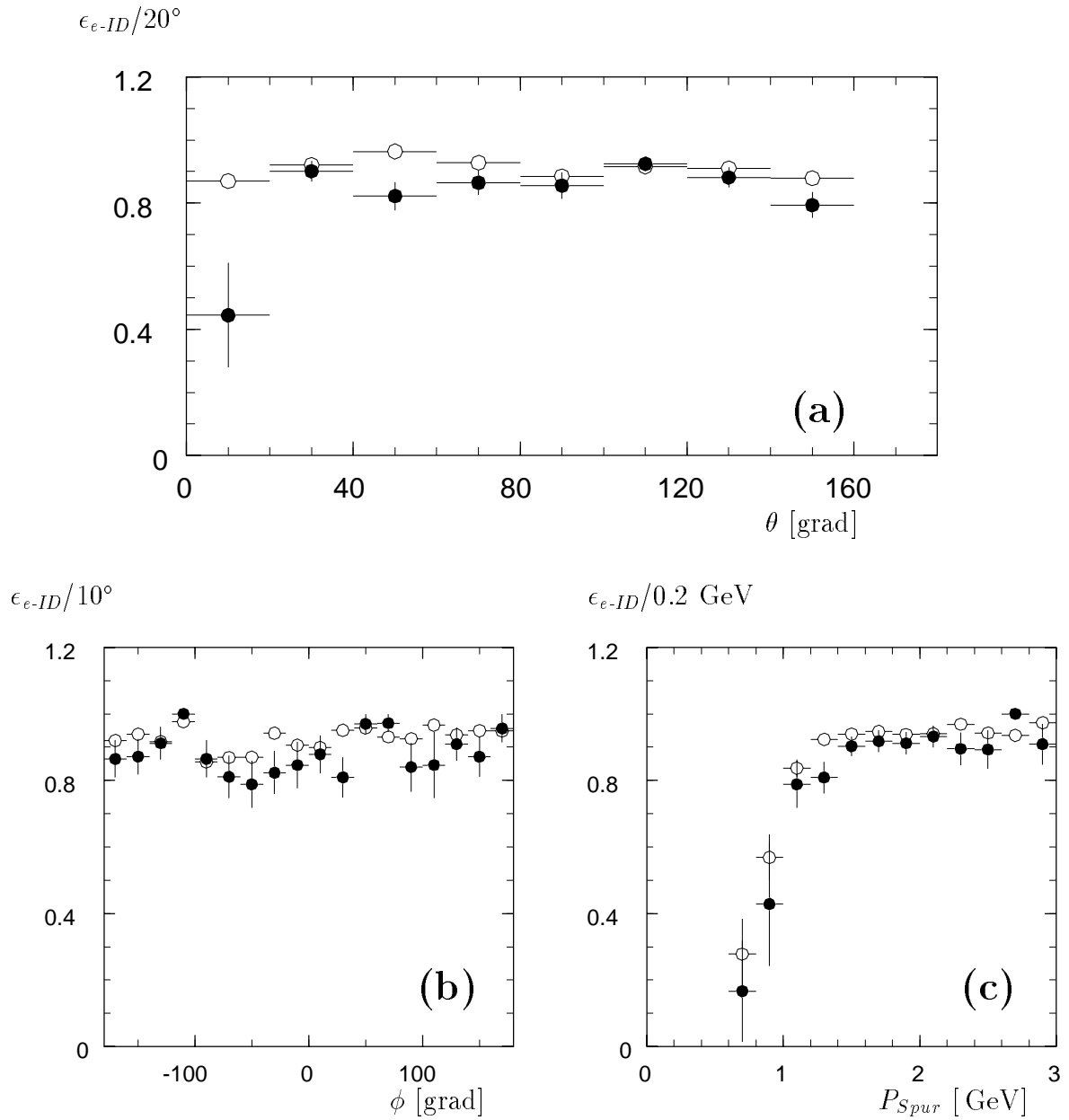
Abbildung 5.3: Elektronnachweiswahrscheinlichkeit in Abhängigkeit vom Polarwinkel (a), dem Azimutalwinkel (b) und dem Impuls (c) der Spur. Die ausgefüllten Punkte stehen für die Daten und die Kreise für die Monte-Carlo-Simulation.
