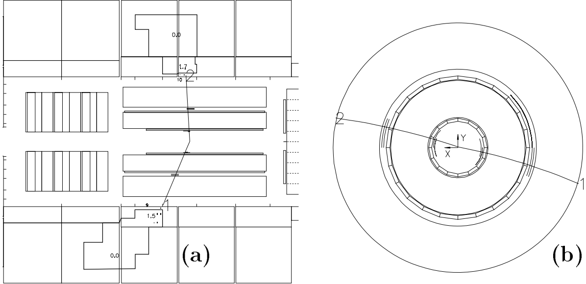
Abbildung 4.1: Abbildungen (a) und (b) erläutern die Funktionsweise des Triggers. (a) zeigt ein J/\psi \rightarrow e^+e^- -Ereignis in der rz -Ansicht. Das e^+e^- -Paar löst Signale in den Proportionalkammern aus, die die Ray-Information für den z -Vertex-Trigger liefern. Weiterhin sprechen die Segmente des Kalorimetertriggers an, die ein weiteres Triggererelement liefern. In (b) wird die MWPC-Information in der r\phi -Projektion gezeigt. Die beiden Spuren liegen koplanar zueinander. Dies löst das Triggererelement topo--BR aus.
