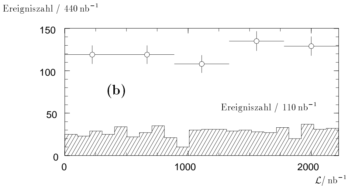
Abbildung 4.8: Abbildung (a) zeigt die integrierte Luminosität über die Datennahmeperiode (obere Kurve). Die untere Kurve ergibt sich nach der Korrektur einzelner Datennahmeperioden, bei denen nicht alle verwendeten Detektorelemente in Betrieb waren. Abbildung (b) zeigt für dieselbe Periode die Anzahl von selektierten e^+e^- -Paaren pro 440 \text{ nb}^{-1} . Das überlagerte Histogramm zeigt die gleichen Daten mit einer kleineren Intervallbreite.
