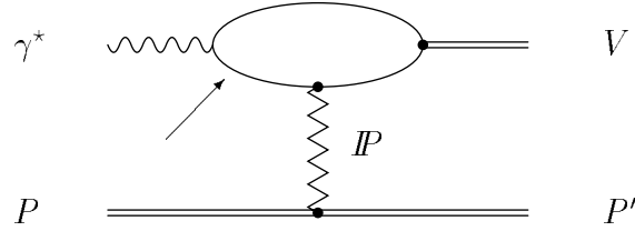
Abbildung 1.8: Diagramm für \gamma^* p \rightarrow V p bei großem Q^2 . Die mit dem Pfeil gekennzeichnete Quarklinie ist weit von der Massenschale entfernt (Abb. aus [Don87]).
