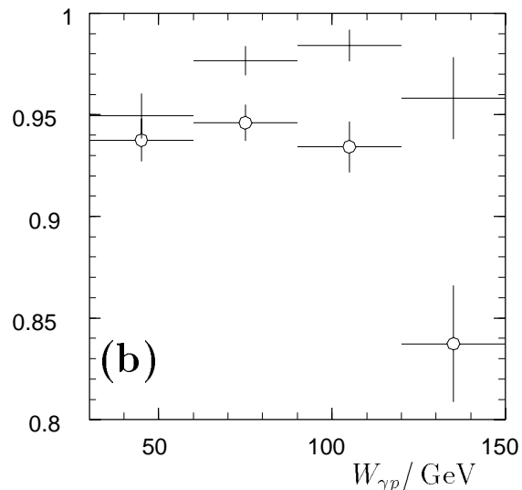
Abbildung 5.13: Abbildung (a) zeigt in Abhängigkeit von W_{\gamma p} die Akzeptanz für protoninelastische Ereignisse durch die Selektion NV , die Schauerpartikel aus der Protondissoziation nachweist. Abbildung (b) zeigt den Einfluß der Multiplizitätsbedingung, die nur die beiden Spuren des e^+e^- -Paares im Spurkammersystem zuläßt, auf den Nachweis von protoninelastischen Ereignissen. Im Monte-Carlo-Modell wird der Fall n = 2 durch Punkte mit Kreisen und n = 2.5 durch die Balken dargestellt.
