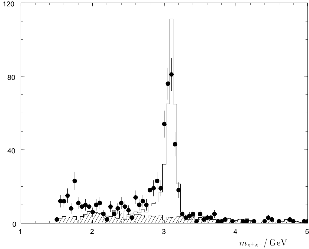
Abbildung 4.7: Die Massenverteilung der e^+e^- -Kandidaten nach Zweispurselection und Elektronerkennung. Die Punkte stehen für die Daten. Das MC-Modell ist den Daten als Histogramm überlagert und auf die Daten im Massenbereich |m - m_{J/\psi}| < 275 \text{ MeV} des J/\psi -Mesons normiert. Die QED-Untergrundereignisse nach sämtlichen Selektionsschnitten sind schraffiert dargestellt. Deren Normierung entspricht der gesammelten Luminosität von \mathcal{L} = 2.1 \text{ pb}^{-1} .
