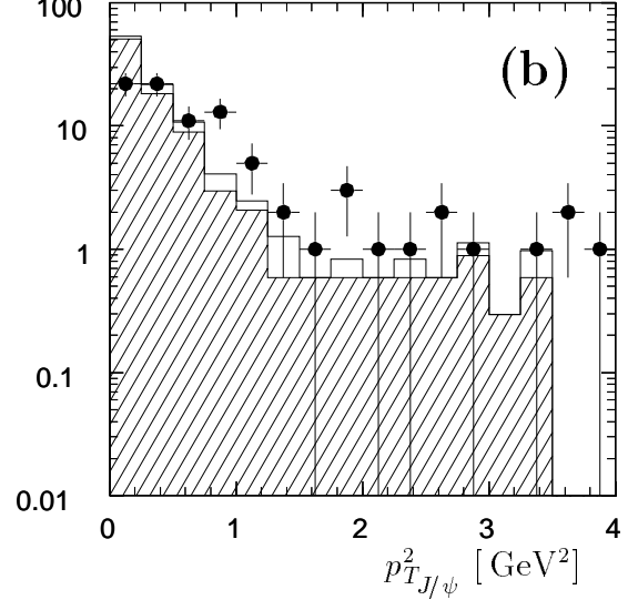
Abbildung 6.3: Abbildung (a) zeigt p_{T,J/\psi}^2 für die Vorwärtsselektion V . Wie in Abbildung 6.2 werden hier Daten und Monte-Carlo-Modell überlagert. Das Histogramm zeigt die Summe aus protonelastischen und inelastischen Ereignissen. Der protoninelastische Anteil ist schraffiert dargestellt. Abbildung (b) zeigt dieselbe Verteilung nach der Selektion NV .
