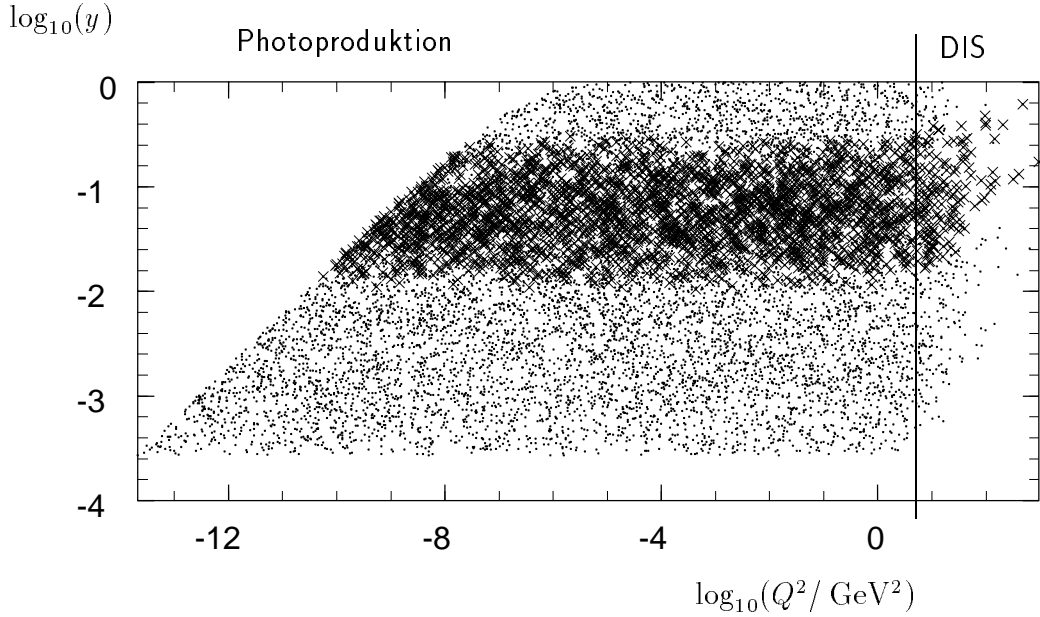
Abbildung 3.1: Korrelation zwischen y und Q^2 der von DIFFVM generierten Ereignisse. Die Ereignisse liegen in der kinematischen Region von Photoproduktion und DIS-Ereignissen. Die mit \times gekennzeichneten Ereignisse erfüllen die Bedingung des Polarwinkelbereichs aus der Abbildung 3.2.
