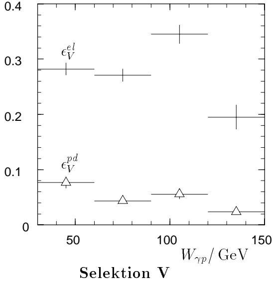
Abbildung 5.14: Detektorakzeptanz in Abhängigkeit von W_{\gamma p} getrennt für protonelastische und protoninelastische Ereignisse. Links sind die Akzeptanzen im Fall der Selektion V und rechts für die Selektion NV abgebildet. Das e^+e^- -Paar muß im Polarwinkelbereich zwischen 20^\circ < \theta < 160^\circ liegen und Q^2 < 4 \text{ GeV}^2 betragen. Der protonelastische Akzeptanzverlauf wird durch Balken und die protoninelastische Akzeptanz durch Dreiecke dargestellt.
