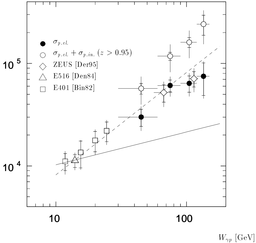
Abbildung 6.1: Die in dieser Analyse ermittelten Wirkungsquerschnitte im Vergleich zu anderen Messung in Abhängigkeit von W_{\gamma p} . Die protonelastischen Messungen werden durch ausgefüllte Kreise gekennzeichnet. Die Summe von elastischer und protoninelastischer Messung für (z > 0.95) bilden die nicht ausgefüllten Kreise. Die durchgezogene Linie zeigt das Ansteigen von \sigma_{\gamma p}(W_{\gamma p}) \propto W_{\gamma p}^{4\epsilon} mit \epsilon = 0.081 . Für die gestrichelte Linie wurde \epsilon auf 0.25 erhöht.
