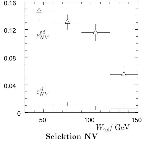
Abbildung 5.14: Detektorakzeptanz in Abhängigkeit von W_{\gamma p} getrennt für protonelastische und protoninelastische Ereignisse. Links sind die Akzeptanzen im Fall der Selektion V und rechts für die Selektion NV abgebildet. Das e^+e^- -Paar muß im Polarwinkelbereich zwischen 20^\circ < \theta < 160^\circ liegen und Q^2 < 4 \text{ GeV}^2 betragen. Der protonelastische Akzeptanzverlauf wird durch Balken und die protoninelastische Akzeptanz durch Dreiecke dargestellt.
