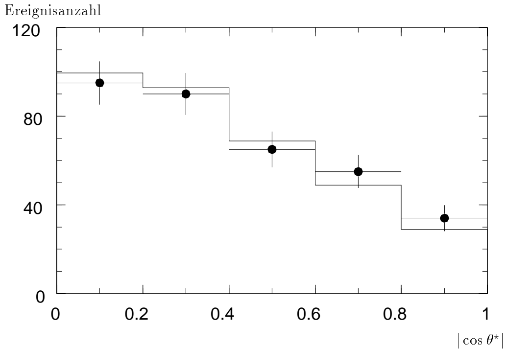
Abbildung 6.4: Vergleich der Zerfallswinkelverteilung für J/\psi -Kandidaten zwischen Daten und Monte-Carlo-Modell, welches als Histogramm überlagert ist.
