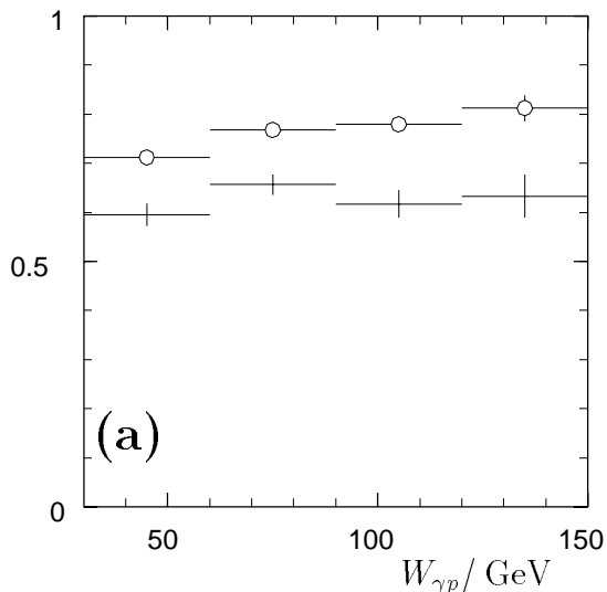
Abbildung 5.13: Abbildung (a) zeigt in Abhängigkeit von W_{\gamma p} die Akzeptanz für protoninelastische Ereignisse durch die Selektion NV , die Schauerpartikel aus der Protondissoziation nachweist. Abbildung (b) zeigt den Einfluß der Multiplizitätsbedingung, die nur die beiden Spuren des e^+e^- -Paares im Spurkammersystem zuläßt, auf den Nachweis von protoninelastischen Ereignissen. Im Monte-Carlo-Modell wird der Fall n = 2 durch Punkte mit Kreisen und n = 2.5 durch die Balken dargestellt.
