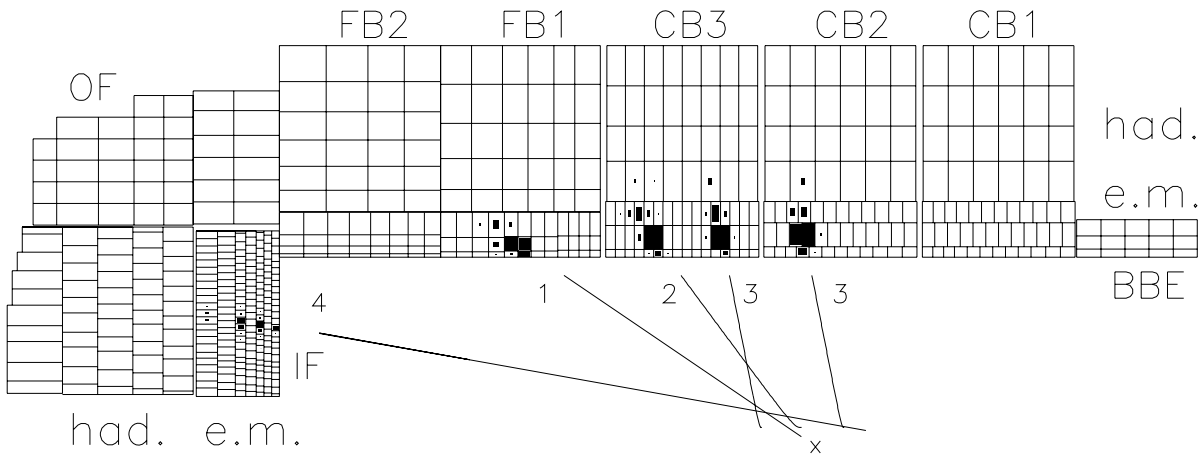
FIG. 4.8: Couches et cellules du LAr, avec des exemples de gerbes formées par des électrons.
