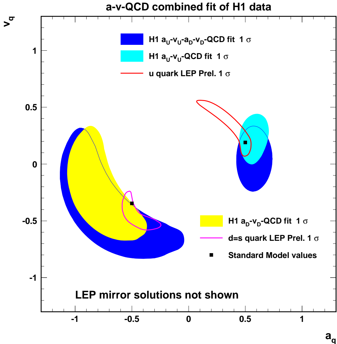
FIG. 8.10: Résultat des ajustements combinés QCD- a_q - v_q . Les résultats des trois ajustements différents sont montrés : lorsque les quatre couplages sont libres, et lorsque les couplages du U ou du D seulement sont libres. Les résultats de LEP pour les quarks légers sont montrés pour comparaison.
