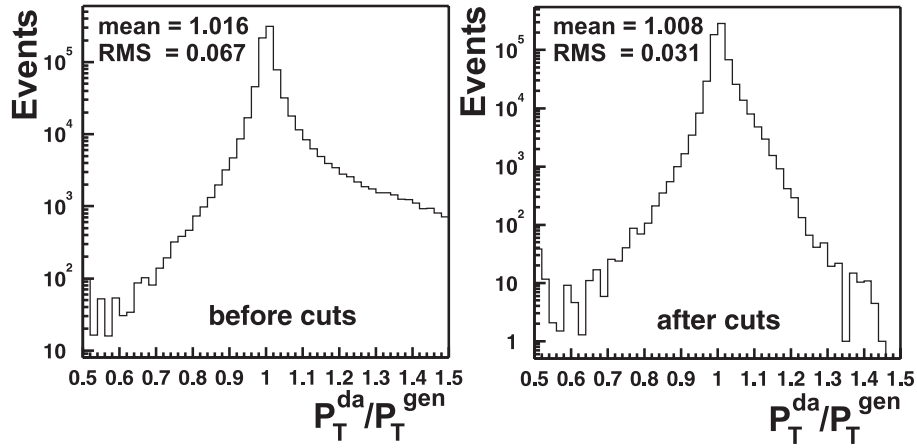
FIG. 5.20: Distributions P_T^{da}/P_T^{gen} avant et après avoir appliqué les sélections de qualité de la mesure de l'impulsion transverse double angle.
