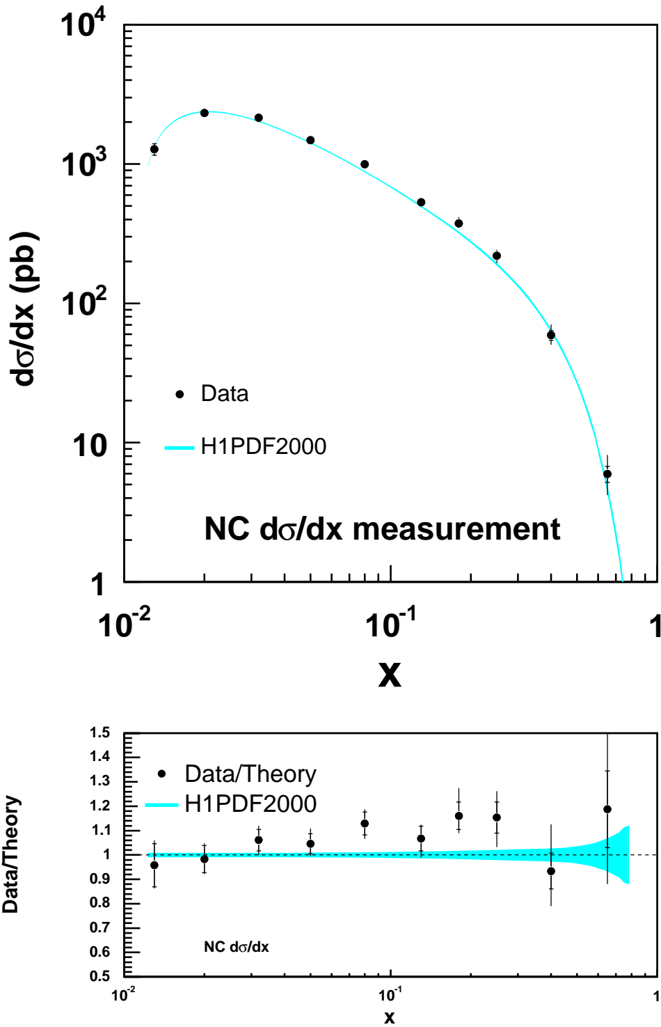
FIG. B.5: Sections efficaces d\sigma/dx ( y < 0,9 , Q^2 > 1000 GeV 2 ) pour la période L. Les bandes et barres d'erreurs sont définies comme sur la figure B.1.
