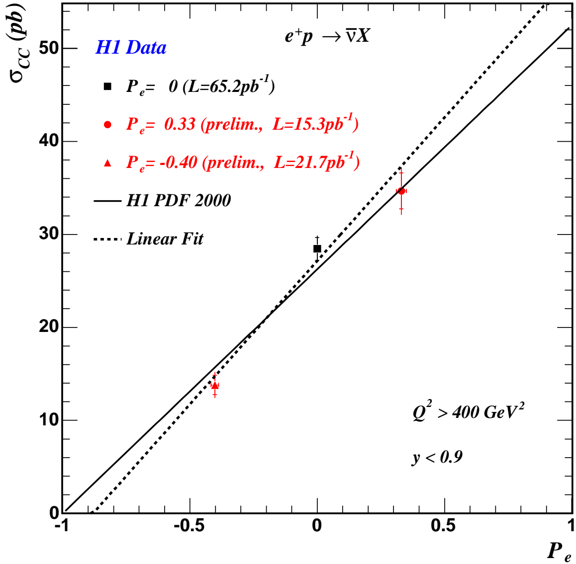
FIG. 7.15: Mesure de la section efficace e^+p CC en fonction de la polarisation P_e . Les données sont comparées à la prédiction de l'ajustement H1PDF2000. La ligne en pointillés est le résultat d'un ajustement aux données.
