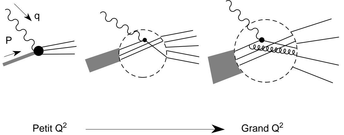
FIG. 2.8: Illustration de la brisure de l'invariance d'échelle introduite par QCD. Lorsque l'on augmente le Q^2 , on distingue des structures de plus en plus petites dans le proton.
