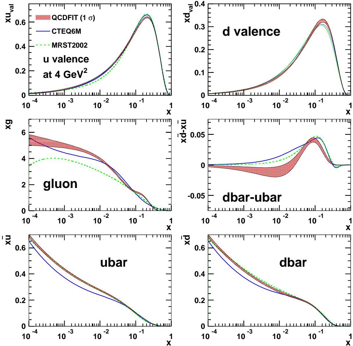
FIG. 9.4: Densités de partons à Q_0^2 = 4 \text{ GeV}^2 . L'aire hachurée correspond à la bande d'erreur à 1\sigma pour les pdfs. La ligne pleine correspond aux pdfs de CTEQ6 et la ligne pointillée correspond aux pdfs de MRST02.
