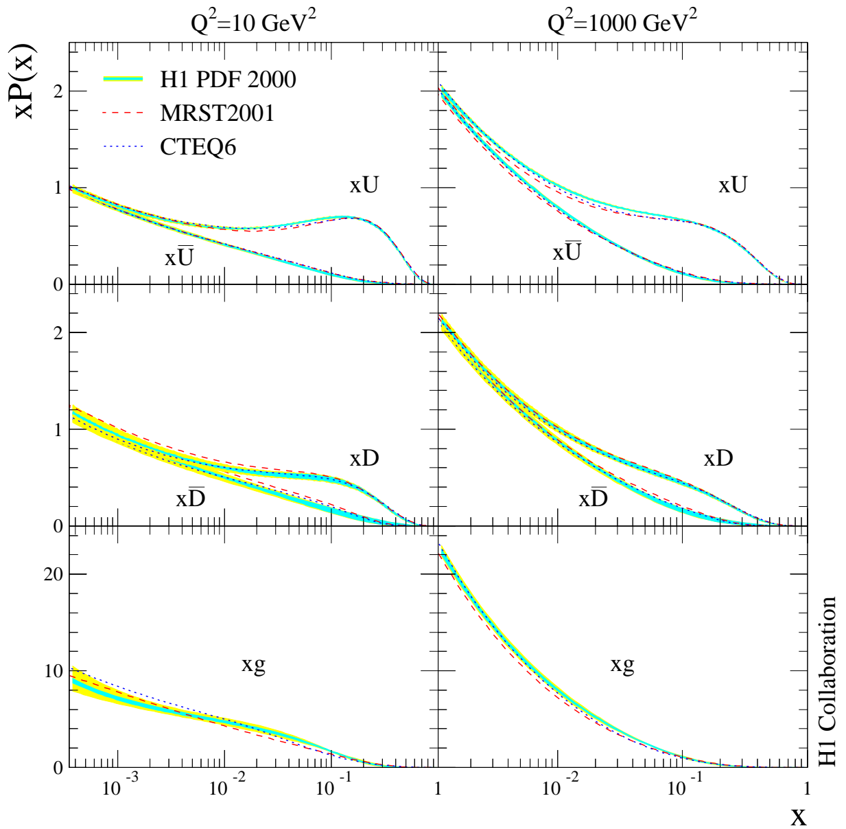
FIG. 8.3: Distributions de partons déterminées dans l'ajustement des données de H1 seul à Q^2 = 10 \text{ GeV}^2 et Q^2 = 1000 \text{ GeV}^2 , comparées aux pdfs de CTEQ et MRST.
