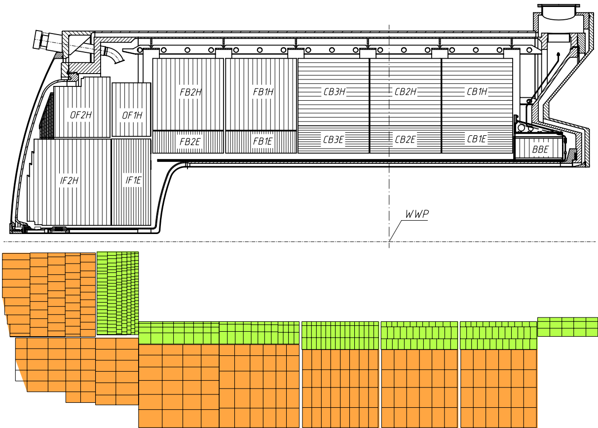
FIG. 4.6: Section longitudinale du calorimètre à Argon liquide. La partie supérieure montre la structure en roues avec l'orientation des plaques d'absorbeur. La structure en cellules est montrée sur la partie inférieure.
