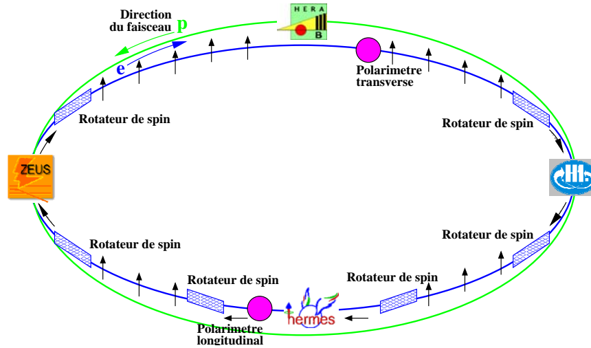
FIG. 4.2: Schéma du collisionneur HERA pour la phase HERAII.
