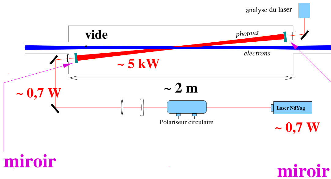
FIG. 4.27: Schéma de principe de la mise en œuvre de POLCA autour du faisceau d'électrons.
