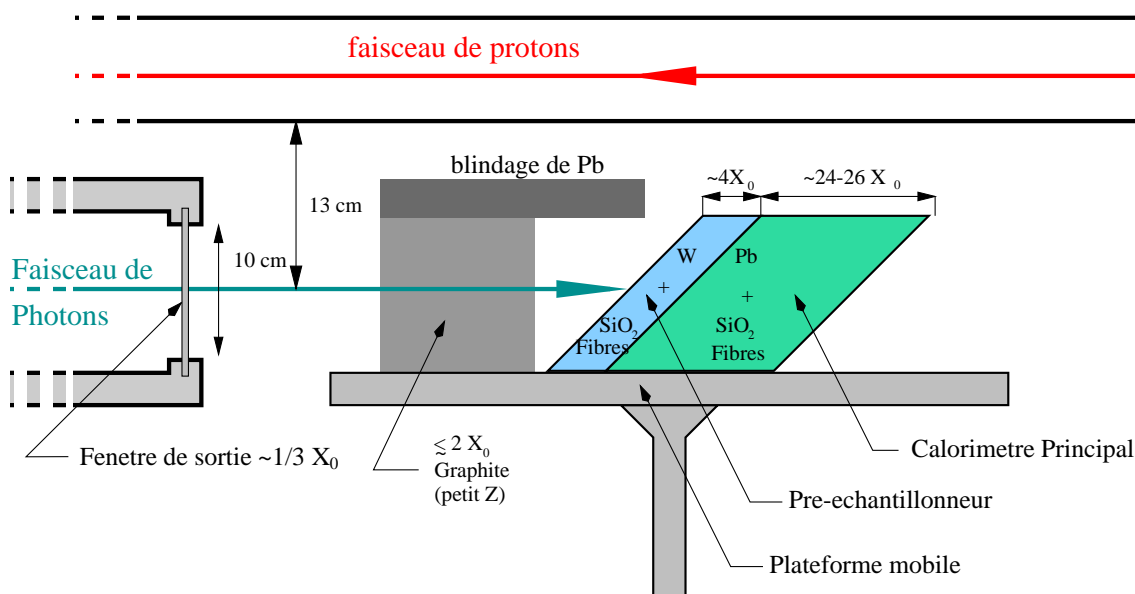
FIG. 4.20: Schéma du luminomètre dans le tunnel dans le plan y - z .
