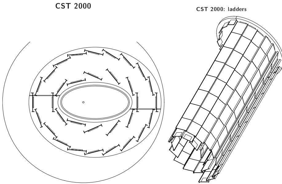
FIG. 4.15: A gauche, vue de la CST dans le plan x - y . A droite, vue tridimensionnelle de l'organisation des plans de détection.
