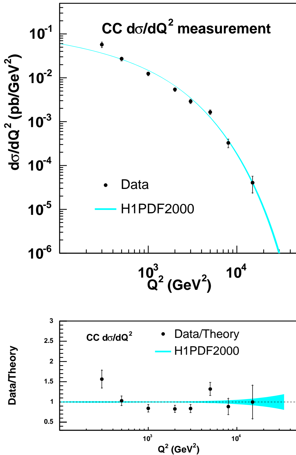
FIG. B.10: Sections efficaces d\sigma/dQ^2 ( y < 0,9 ) pour la période L. Les bandes et barres d'erreurs sont définies comme sur la figure B.8.
