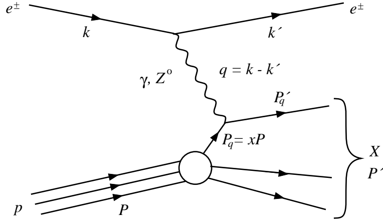
FIG. 2.2: Diffusion entre un lepton chargé et un hadron. Les quadrivecteurs sont définis sur la figure.
