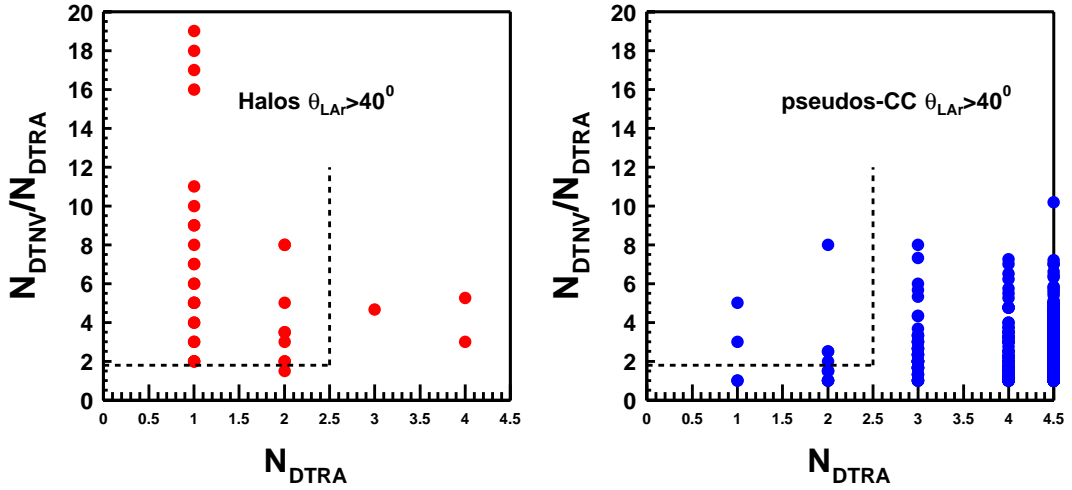
FIG. 7.2: Distribution des événements pseudo-CC et des halos dans le plan \theta_{LAr}, \varphi_{LAr} et N_{DTNV}/N_{DTRA}, N_{DTRA} . La sélection effectuée est indiquée par le trait pointillé.
