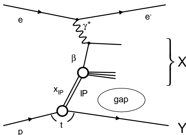
FIG. 2.13: Interaction du photon virtuel avec un poméron, produisant un gap de pseudo-rapacité entre le proton diffusé et l'état final hadronique.
