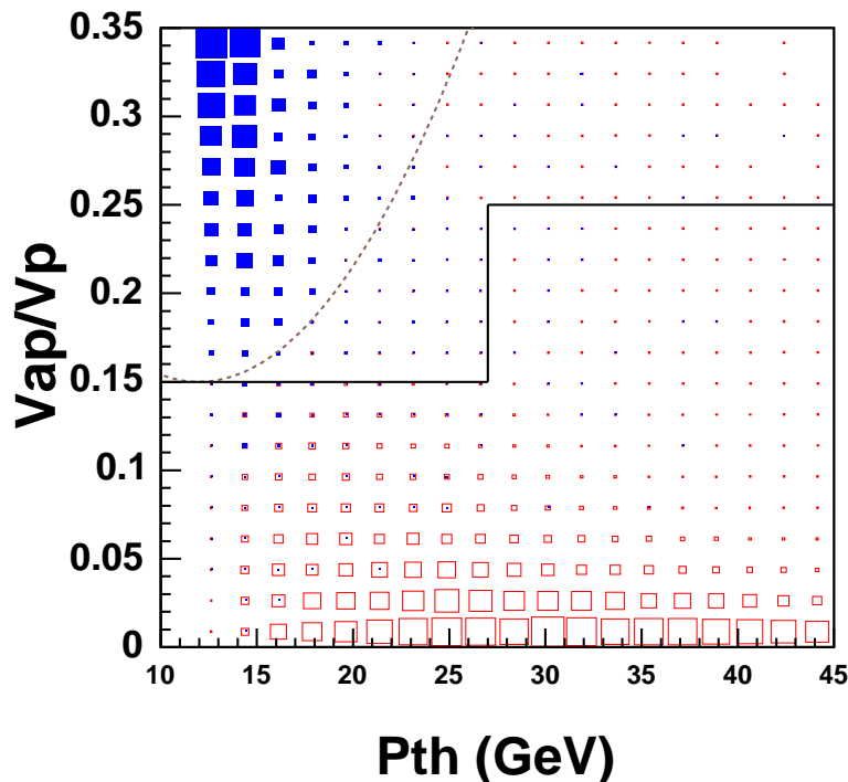
FIG. 7.5: Distribution des événements CC (carrés blancs à bords rouges) et des événements \gamma p (carrés bleus pleins) dans le plan pt_h, V_{ap}/V_p . La ligne noire représente la coupure rectangulaire, et la ligne pointillée la coupure parabolique.
