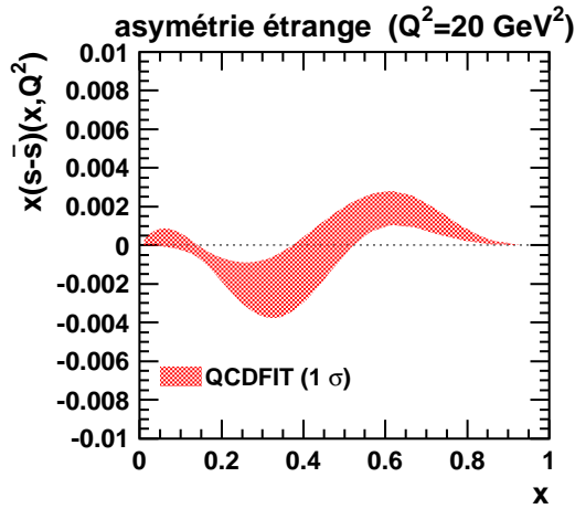
FIG. 9.9: Asymétrie de la mer étrange obtenue en utilisant les données de CDHSW et les données de CCFR.
