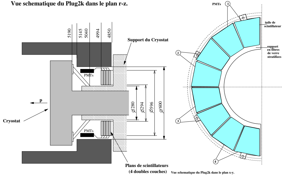
FIG. 4.10: A gauche, coupe longitudinale du Plug2k. A droite, vue de la moitié tuiles de scintillateur dans le plan transverse.
