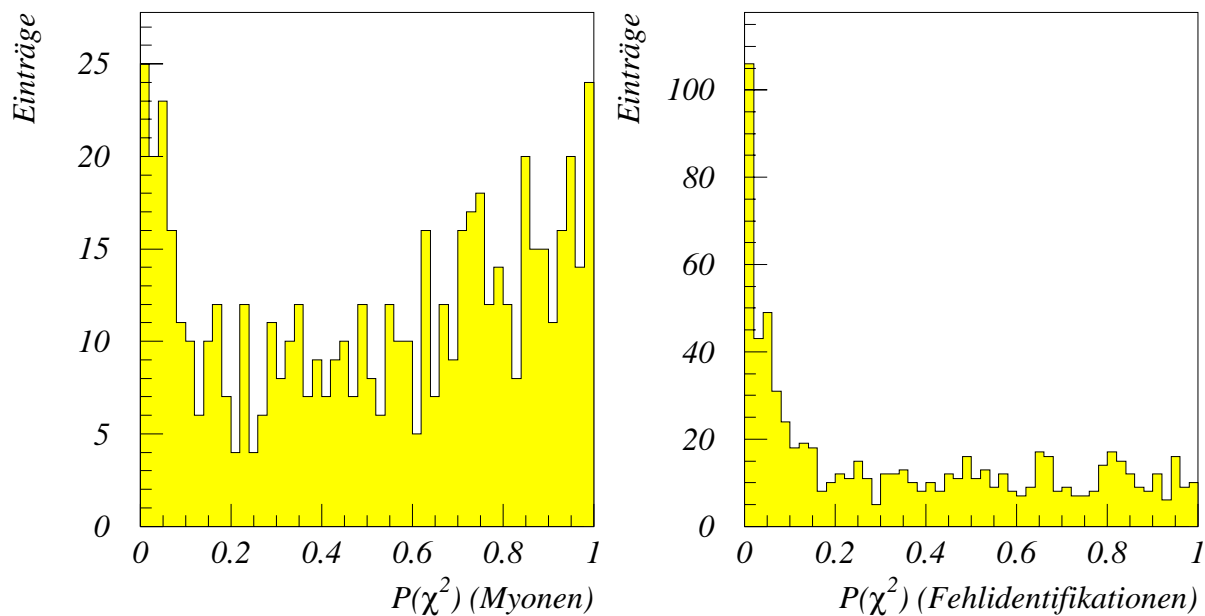
Abbildung 11: Verbindungswahrscheinlichkeit P(\chi^2) für Myonen (links) und für Fehlidentifikationen (rechts)
