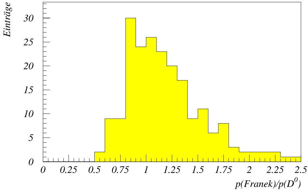
Abbildung 25: Verhältnis von genähertem zu tatsächlichem D^0 -Impuls in der Franek-Methode
