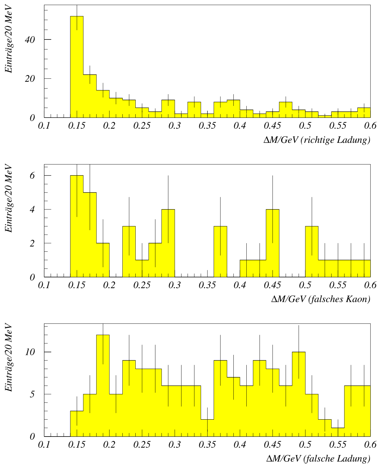
Abbildung 31: Pseudo- \Delta M -Verteilungen im Datensatz DSSIM für die verschiedenen Klassen von Ladungskombinationen
