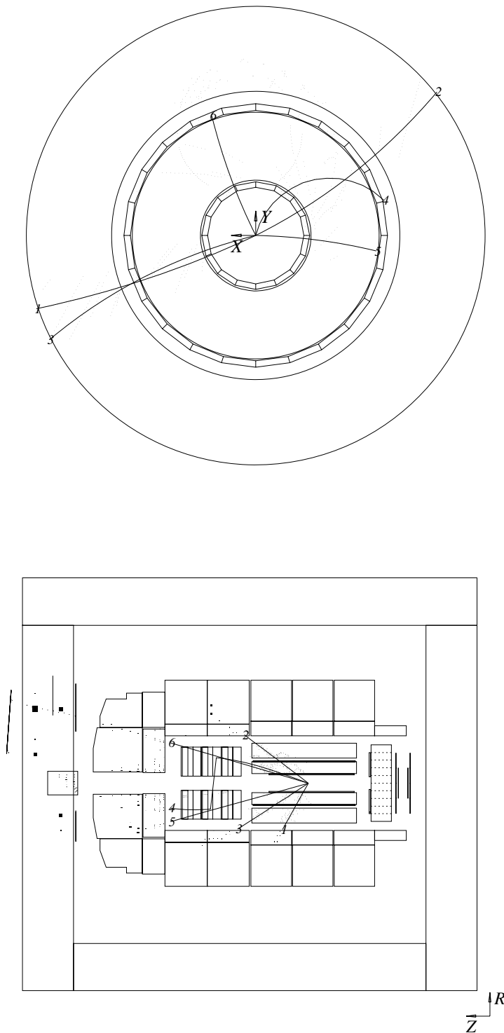
Abbildung 30: Ein Photon-Gluon-Fusionsereignis mit einem Zerfall D^{*-} \rightarrow \bar{D}^0 \pi^- \rightarrow (K^+ \mu^- \bar{\nu}_\mu) \pi^-
