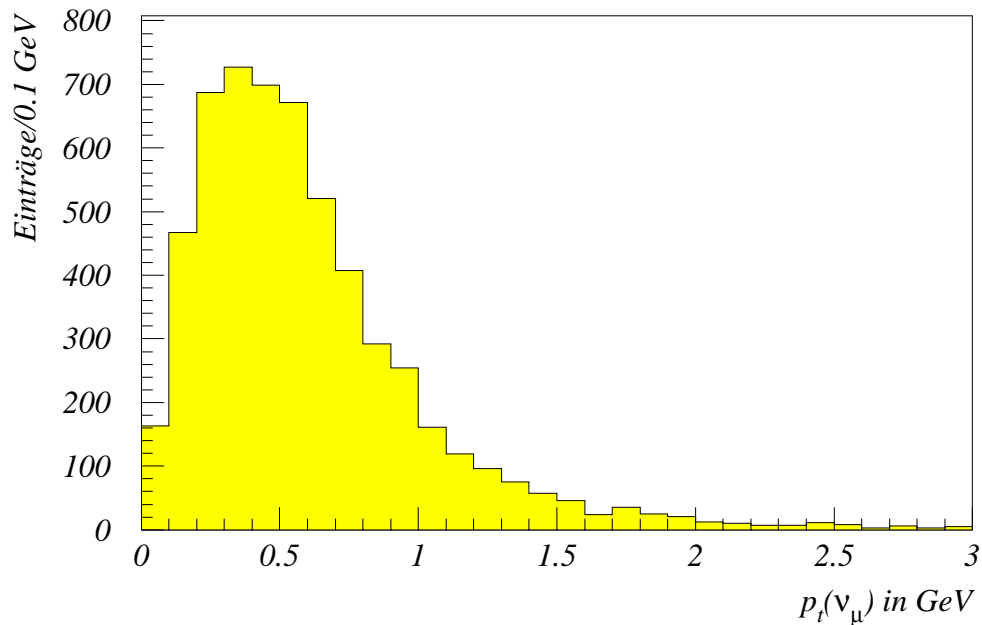
Abbildung 19: Transversalimpuls der Neutrinos aus dem Zerfall D^0 \rightarrow K^- \mu^+ \nu_\mu
