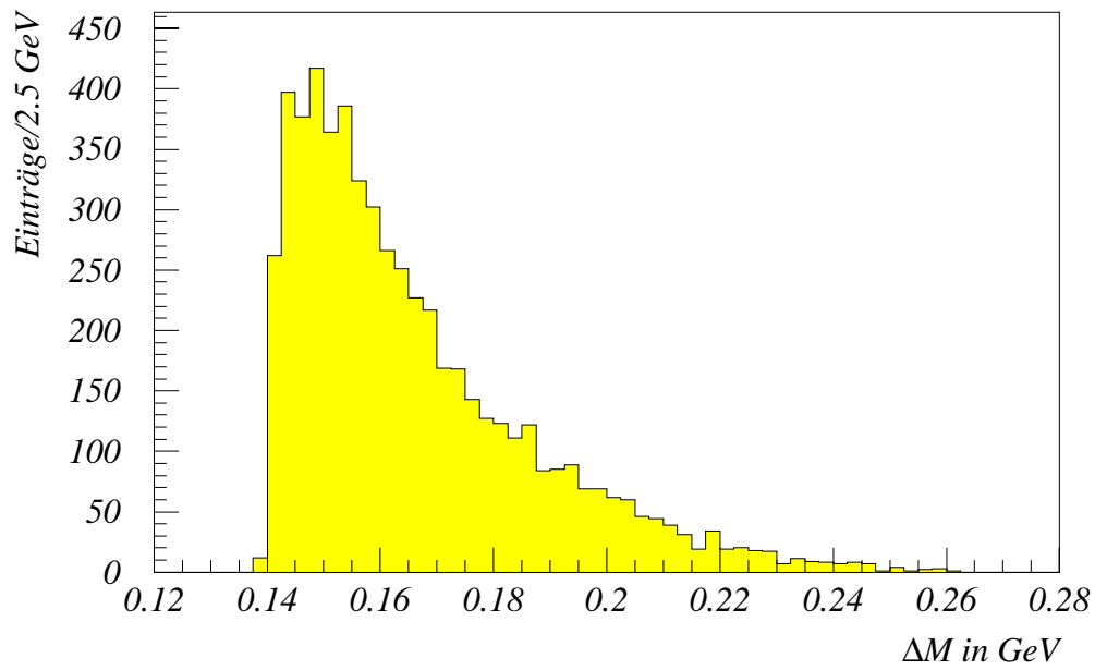
Abbildung 6: Pseudo- \Delta M -Verteilung im Zerfall D^{*+} \rightarrow D^0 \pi^+ \rightarrow (K^- \mu^+ \nu_\mu) \pi^+ auf Monte-Carlo-Ebene
