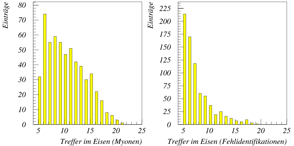
Abbildung 13: Anzahl der Treffer im instrumentierten Eisen für Myonen (links) und für Fehlidentifikationen (rechts)
