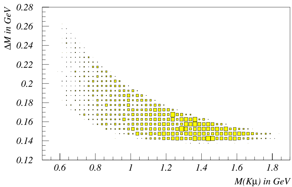
Abbildung 7: Pseudo- \Delta M -Verteilung in Abhängigkeit von M(K^- \mu^+) auf Monte-Carlo-Ebene
