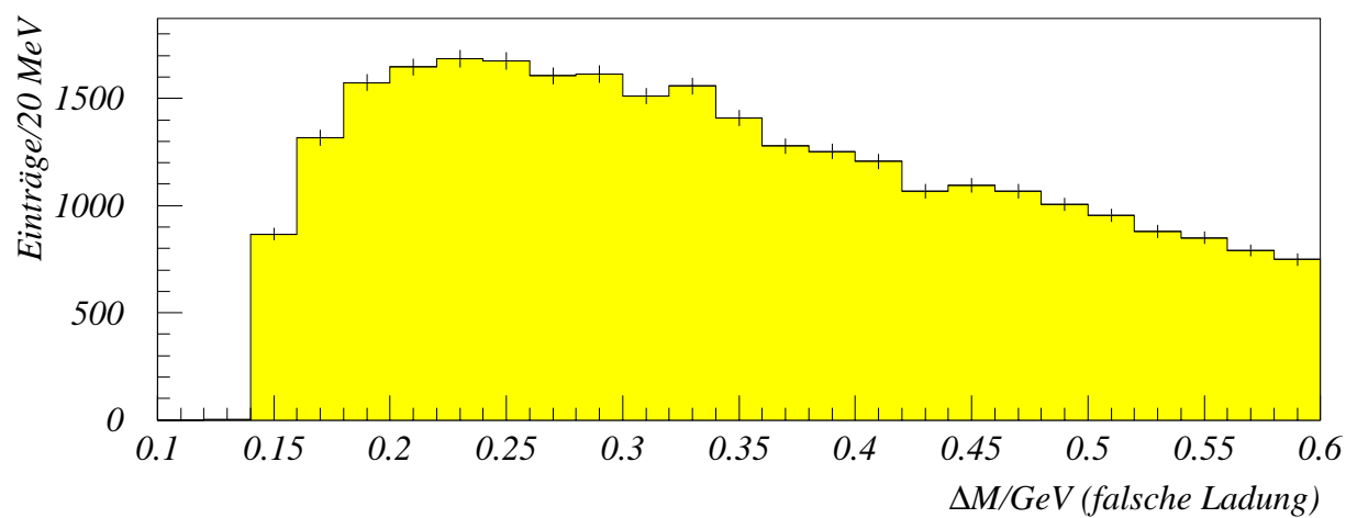
Abbildung 36: Pseudo- \Delta M -Verteilungen im Datensatz DST4 für die verschiedenen Klassen von Ladungskombinationen
