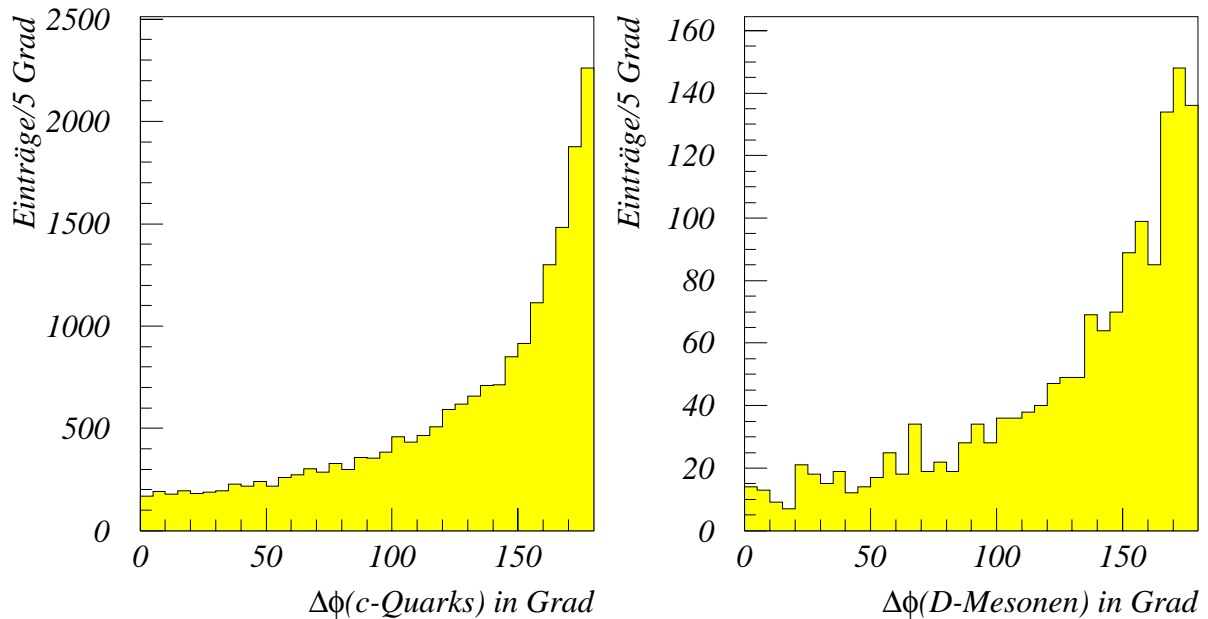
Abbildung 9: Azimutalwinkeldifferenz für c\bar{c} -Paare (links) und D^{*+}D^{*-} -Paare (rechts)
