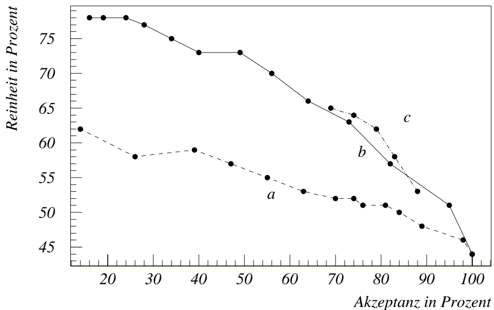
Abbildung 12: Reinheit über Akzeptanz für einen Schnitt in der Verbindungswahrscheinlichkeit (a), für einen Schnitt in der Anzahl der Treffer im instrumentierten Eisen (b) und für einen kombinierten Schnitt (c)
