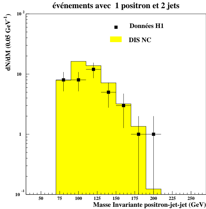
Figure 5.21: Masse invariante positron-jet-jet pour les candidats e^* \rightarrow eZ_{\rightarrow q\bar{q}} et \nu^* \rightarrow eW_{\rightarrow q\bar{q}} . Les carrés correspondent aux données et l'histogramme grisé à l'estimation du bruits de fond normalisé à la luminosité.
