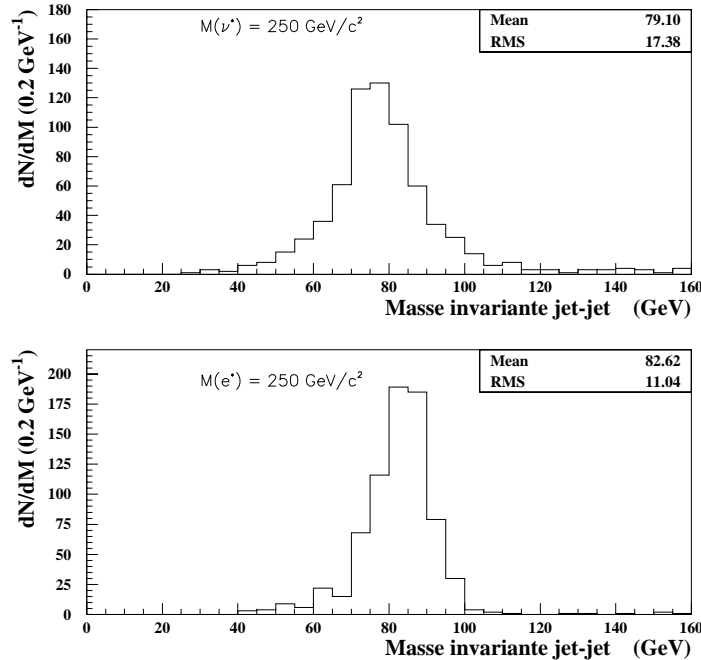
Figure 5.17: Masse invariante jet-jet pour le signal e^* \rightarrow eZ_{\rightarrow q\bar{q}} et \nu^* \rightarrow eW_{\rightarrow q\bar{q}} généré à une masse de 250 \text{ GeV}/c^2 .
