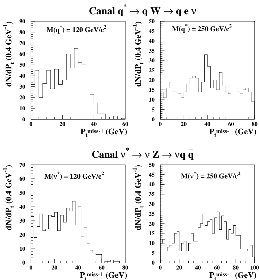
Figure 5.27: Distributions de l'énergie transverse manquante perpendiculaire pour les canaux \nu^* \rightarrow \nu Z \rightarrow \nu q \bar{q} et q^* \rightarrow q W \rightarrow q e \nu .
