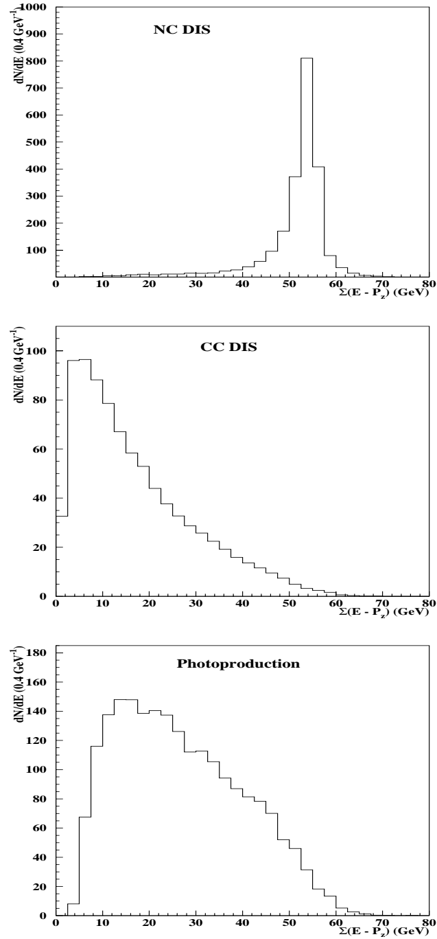
Figure 5.1: Distributions de l’énergie longitudinale \Sigma_i(E_i - P_{z_i}) mesurée dans le calorimètre à argon liquide pour les processus Monte-Carlo Courant Neutre, Courant Chargé et Photoproduction, et normalisées à la luminosité de l’expérience.
