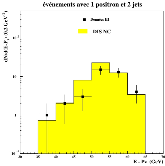
Figure 5.19: Energie longitudinale \sum_i(E_i - P_{z_i}) des candidats sélectionnés pour l'étude des canaux e^* \rightarrow eZ_{\rightarrow q\bar{q}} et \nu^* \rightarrow eW_{\rightarrow q\bar{q}} . Les données sont représentées par les carrés et le bruit de fond par l'histogramme grisé.
