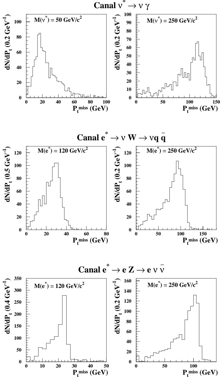
Figure 5.26: Distributions de l'énergie transverse manquante pour les canaux \nu^* \rightarrow \nu \gamma , e^* \rightarrow \nu W \rightarrow \nu q \bar{q} et e^* \rightarrow e Z \rightarrow e \nu \bar{\nu} .
