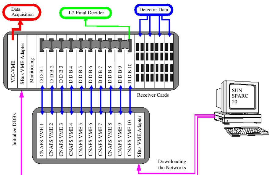
Abbildung 4.2: Übersicht über das L2 Trigger System des H1-Detektors.
