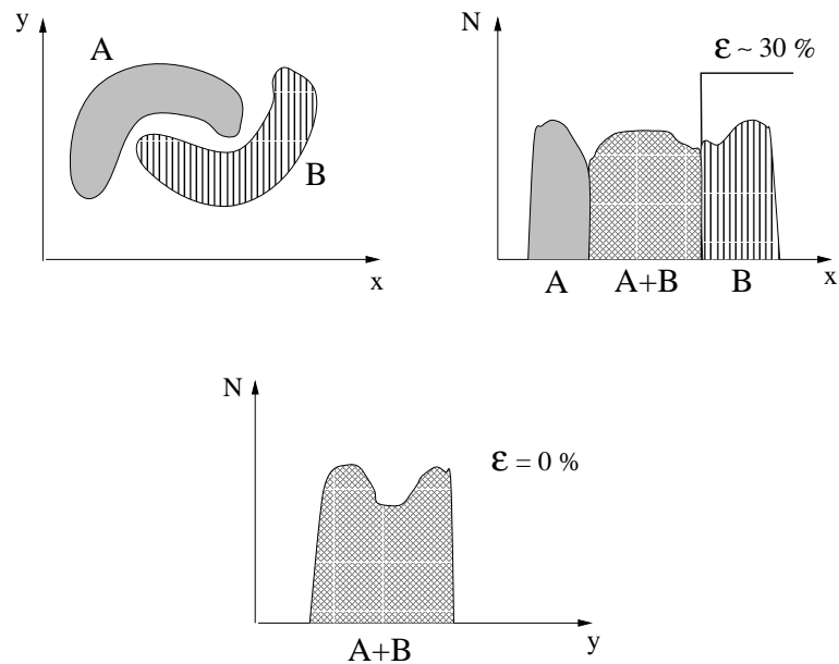
Abbildung 4.3: Beispiel: Die Bereiche der beiden Klassen A und B sind im zwei-dimensionalen Raum separabel. Durch die Beschränkung der Variablen x bzw. y ist keine vollständige Trennung der Klassen möglich.
