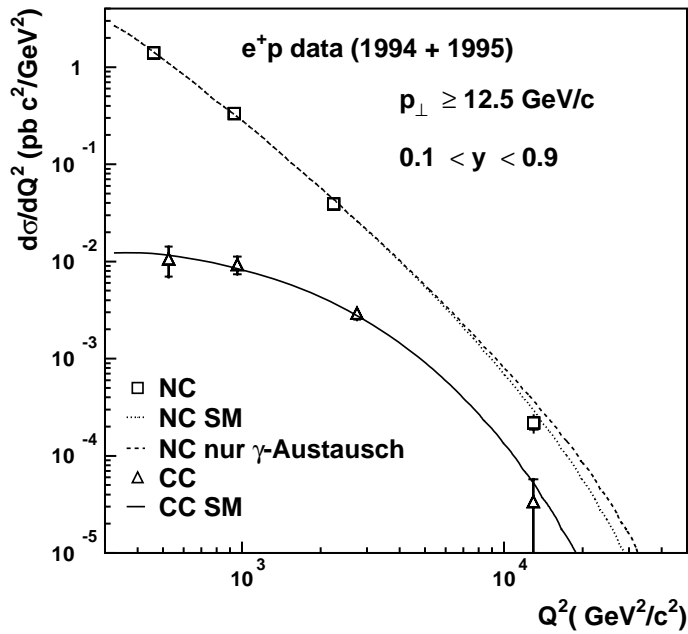
Abbildung 2.2: Gezeigt ist ein Vergleich des gemessenen d\sigma/dQ^2 -Wirkungsquerschnitts des geladenen Stroms und des neutralen Stroms mit der theoretischen Vorhersage des Generators HERACLES unter Verwendung der Partondichte MRSH [MRS93] für den geladenen Strom (durchgezogene Linie) und dem neutralen Strom (gepunktete Linie). Die unterbrochene Linie zeigt die theoretische Vorhersage für den Prozeß des neutralen Stroms unter der Annahme, daß nur virtuelle Photonen ausgetauscht würden. Aus [Mar97].
