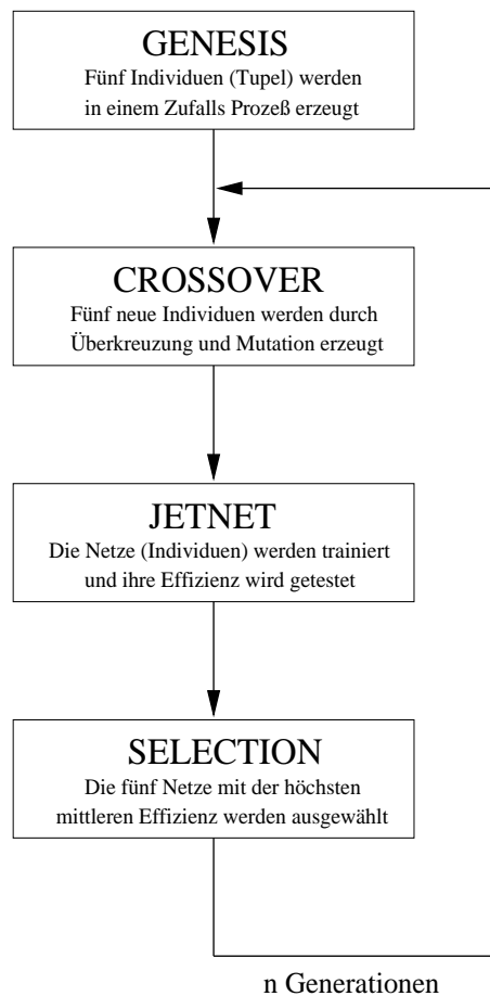
Abbildung 6.2: Darstellung der einzelnen im Optimierungsprozess ablaufenden Programmschritte
