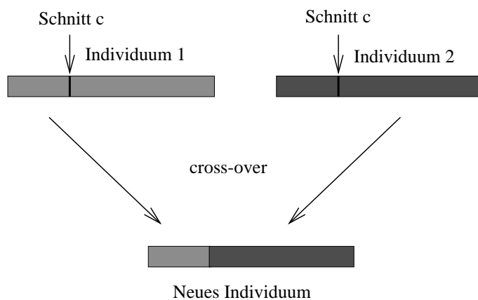
Abbildung 4.7: Funktionsweise des Rekombinationoperators
