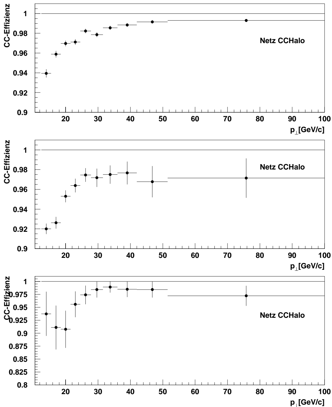
Abbildung 6.17: Die Effizienz der CC-Erkennung des Netzes CCHalo in Abhängigkeit vom Transversalimpuls p_{\perp} . In der oberen Abbildung beim Test mit dem Monte-Carlo Datensatz CCMC in der Mitte beim Test mit den Pseudo-CC Ereignissen des Satzes PSCC und in der unteren Abbildung mit dem CC-Datensatz CCDATA. Man beachte die verschiedenen Effizienzskaalen.
