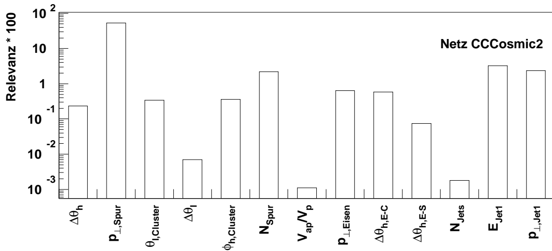
Abbildung 6.22: Die Relevanzen der im Netzwerk CCCosmic verwendeten Eingabevariablen. Die Relevanz ist im logarithmischen Maßstab aufgetragen.
