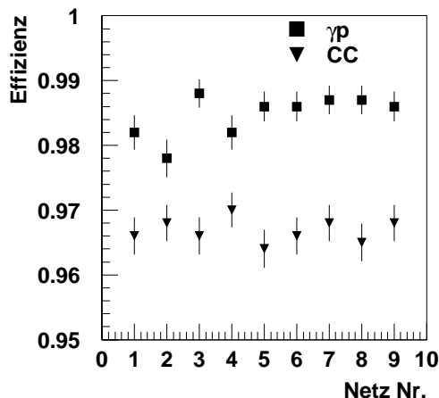
Abbildung 6.12: Die Effizienzen der Netze zur Unterscheidung von CC- und \gamma p -Ereignissen im Vergleich. Die Effizienzen wurden mit den während des Trainings verwendeten Trainings- und Testmustersätzen bestimmt. Angegeben ist der statistische Fehler der Effizienz.
