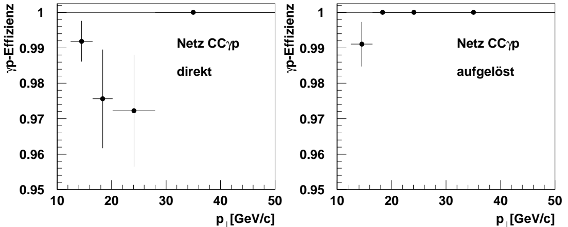
Abbildung 6.15: Die p_{\perp} -Abhängigkeit der Effizienz der \gamma p -Erkennung des Netzes CC\gamma p . Im linken Bild beim Test mit dem Monte Carlo Datensatz \gamma p_{dir3} und rechts beim Test mit \gamma p_{pres3} .
