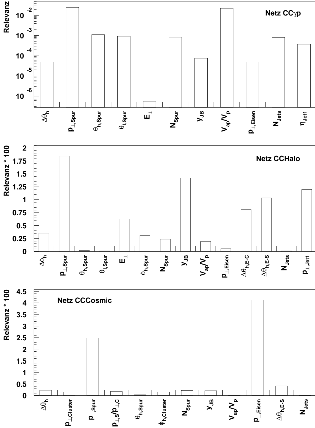
Abbildung 6.21: Die Relevanzen der in den Netzwerken CC\gamma p (oben), CCHalo (Mitte) und CCCosmic (unten) verwendeten Eingabevariablen. Die Relevanz ist in der oberen Abbildung im logarithmischen Maßstab aufgetragen.
