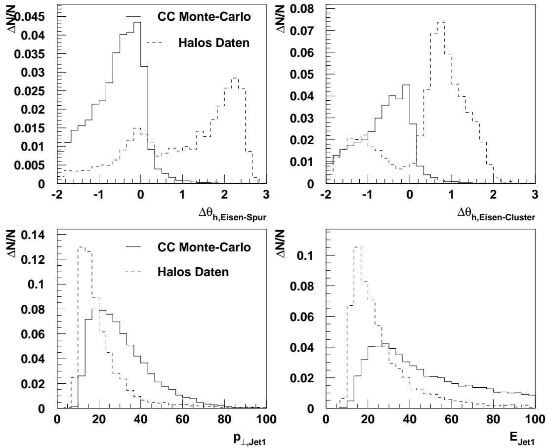
Abbildung 6.8: Verteilungen der möglicher Eingabevariablen \Delta\theta_{Eisen-Spur} und \Delta\theta_{Eisen-Cluster} (oben) sowie p_{\perp,Jet1} und E_{Jet1} (unten) eines neuronalen Netzes zur Erkennung von Halo-Ereignissen.
