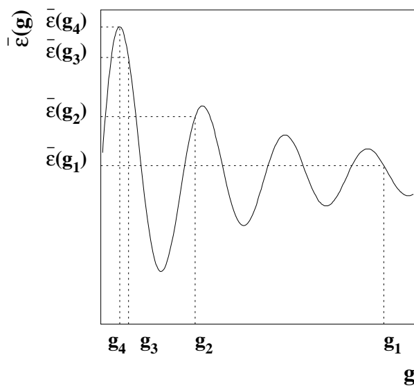
Abbildung 6.4: Dargestellt ist eine hypothetische mittlere Effizienz \bar{\varepsilon}(\mathbf{g}) mit mehreren lokalen Maxima. Die Tupel \mathbf{g} werden in dieser Abbildung durch Werte g auf der Abszissenachse symbolisiert. Der Wert g_i repräsentiert das Tupel mit der höchsten Effizienz in der i -ten Generation.
