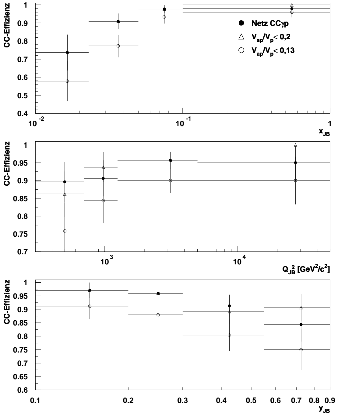
Abbildung 6.27: Die CC-Effizienz des Netzwerkes CC\gamma p in Abhängigkeit von den kinematischen Variablen x_{JB} (oben), Q_{JB}^2 (Mitte) und y_{JB} (unten) beim Test mit dem Datensatz PSCC.
