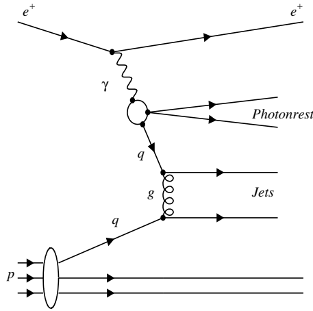
Abbildung 2.4: Feynmandiagramm eines aufgelösten Prozesses
