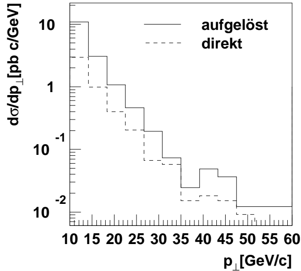
Abbildung 5.5: Abhängigkeit des Wirkungsquerschnitts der direkten und der aufgelösten Photoproduktion vom hadronischen Transversalimpuls p_{\perp} , für Monte-Carlo-Datensätze.
