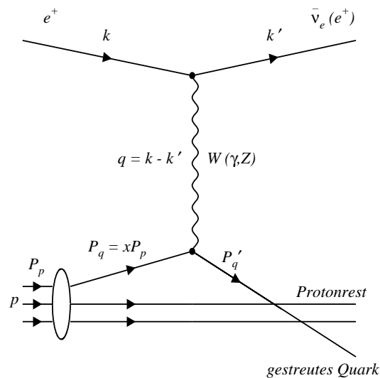
Abbildung 2.1: Feynmandiagramm der tiefunelastischen Positron-Proton-Streuung in niedrigster Ordnung. In der Abbildung werden die Viererimpulse des ein- bzw. auslaufenden Leptons mit k bzw. k' bezeichnet. P_p ist der Viererimpuls des einlaufenden Protons und P_q bzw. P'_q der des einlaufenden bzw. gestreuten Quarks. Der Viererimpulsübertrag wird mit q bezeichnet.
