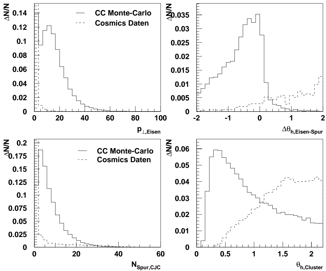
Abbildung 6.7: Die Verteilungen der möglicher Eingabevariablen p_{\perp,Eisen} , \Delta\theta_{h,Eisen-Spur} , N_{Spur,CJC} und \theta_{h,Cluster} eines Netzes zur Trennung von CC-Ereignissen und Cosmics.
