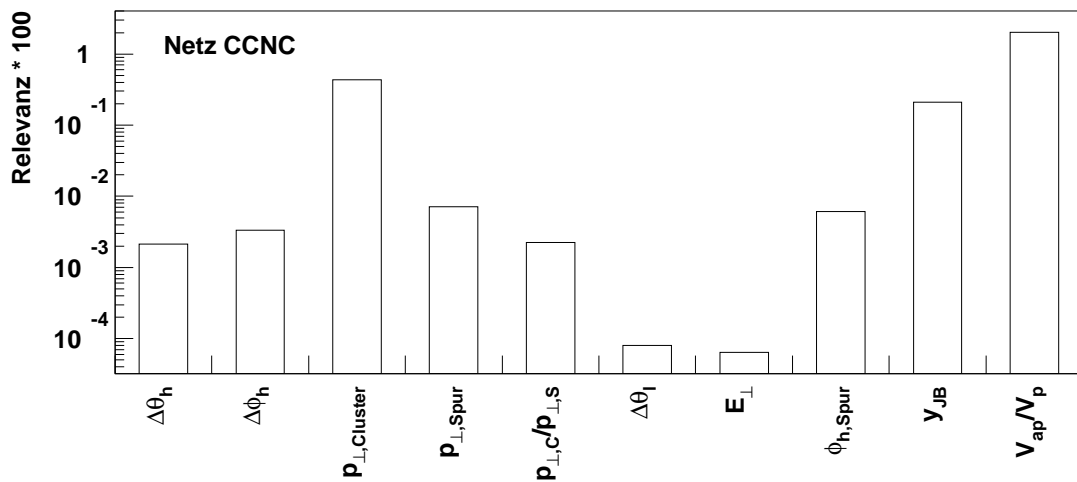
Abbildung 6.23: Die Relevanzen der im Netzwerk CCNC verwendeten Eingabevariablen.
