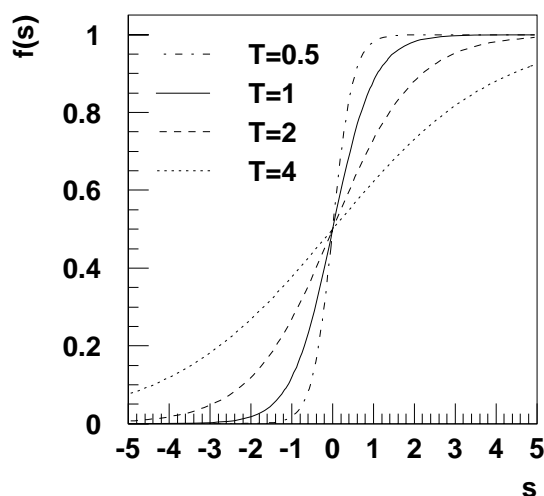
Abbildung 4.6: Die Ausgabefunktion als Funktion der Aktivierung s , bei vier verschiedenen Werten der Temperatur. Für T \rightarrow 0 nähert sie sich der Heaviside-Funktion an.
