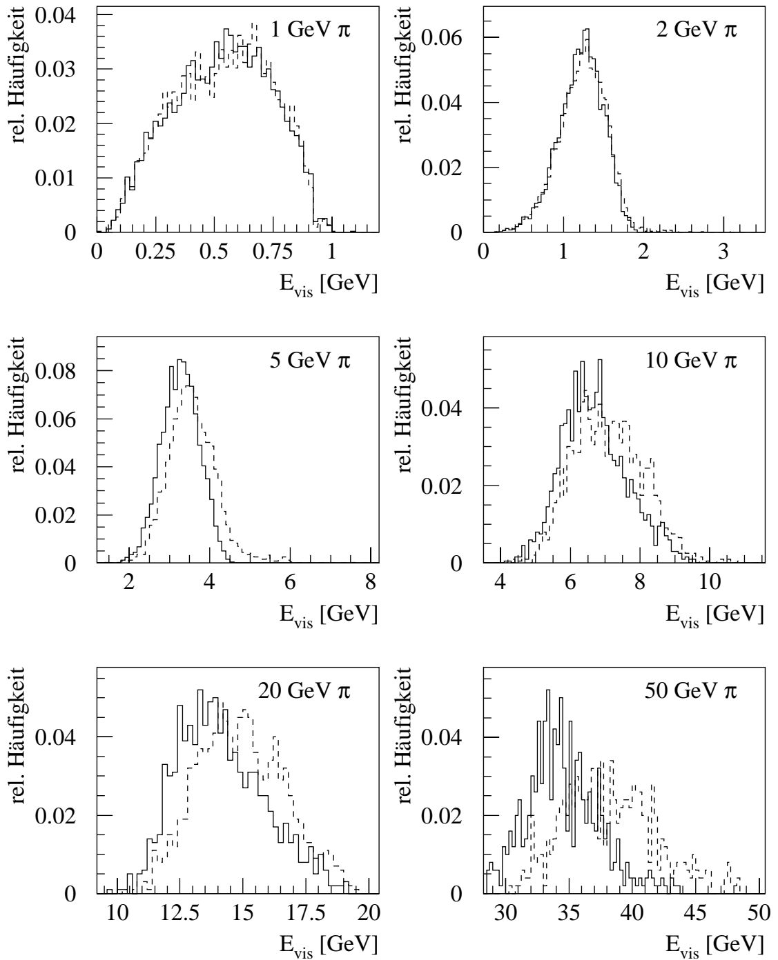
Abbildung A.3: Verteilung der sichtbaren Energie E_{vis} in Pionschauern bei verschiedenen Pionenergien, Simulation mit GHEISHA ohne Korrektur - - - - - und mit Korrektur ———
