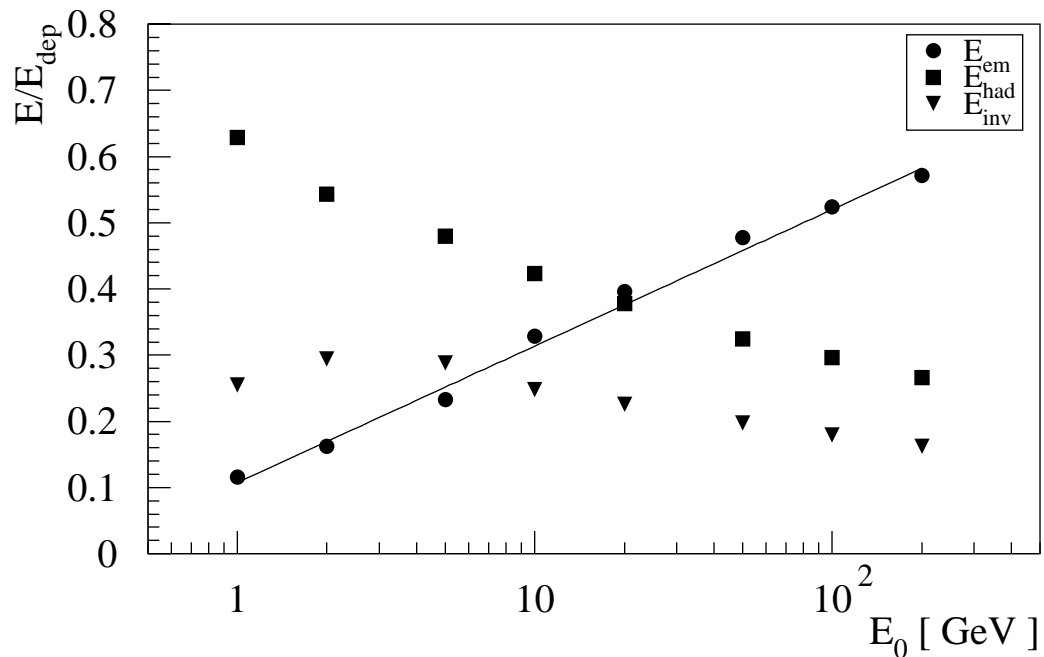
Abbildung 2.7: Aufteilung der deponierten Energie auf die Komponenten eines von Protonen initiierten hadronischen Schauers im Absorber Stahl in Abhängigkeit von der Primärenergie E_0 , eigene Simulation mit CALOR. Die statistischen Fehler sind kleiner als die Symbole.
