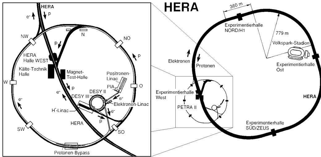
Abbildung 1.1: Skizze des Speicherrings HERA
