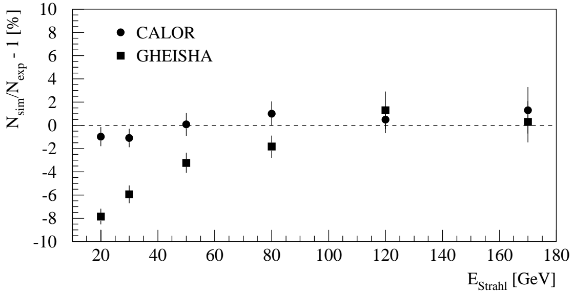
Abbildung 6.9: Relative Abweichung der Anzahl der nach dem Schnitt gegen Rauschen verbleibenden Kanäle in der Simulation von der bei gemessenen Daten.
