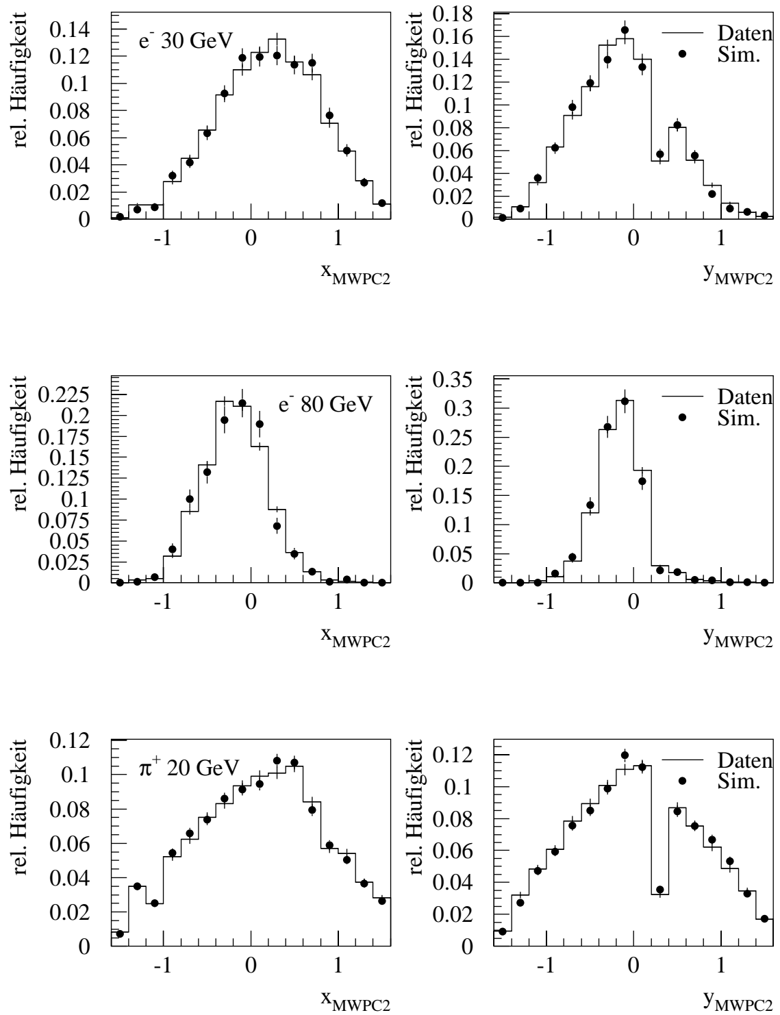
Abbildung 4.11: Gemessene und simulierte Strahlprofile in der MWPC2, x_{MWPC2} und y_{MWPC2} , gemessen in cm.
