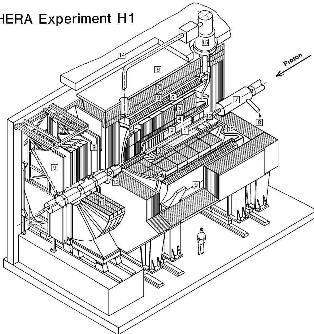
Abbildung 1.2: Perspektivische Ansicht des H1-Detektors
