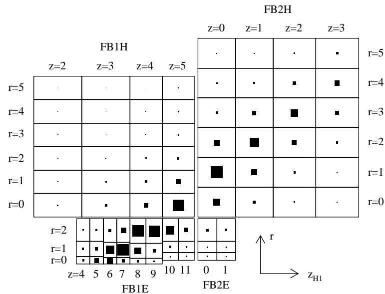
Abbildung 6.2: Verteilung der mittleren Energiedeposition in der r - z_{H1} -Ebene in hadronischen Schauern von 20 GeV Pionen bei Strahlposition 2, Simulation mit CALOR.
