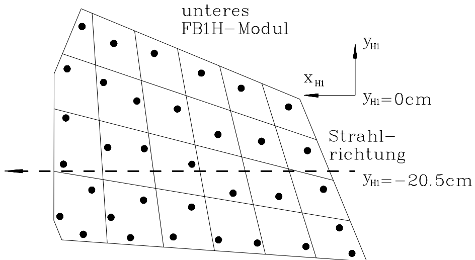
Abbildung 5.8: Strahlposition relativ zu den Auslesekarten des unteren Moduls des FBH-Kalorimeters für Strahlposition 1.
