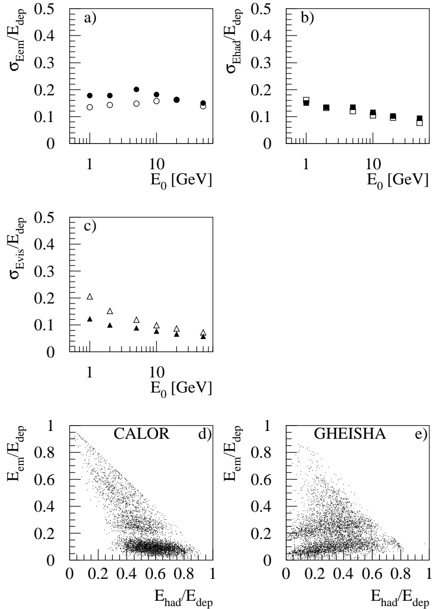
Abbildung 3.2: Fluktuationen a) der elektromagnetischen Komponente \sigma_{E_{em}} , b) der hadronischen Komponente \sigma_{E_{had}} und c) der nachweisbaren Energie \sigma_{E_{vis}} hadronischer Schauer von Pionen in Eisen in Abhängigkeit von der Primärenergie, CALOR volle Symbole, GHEISHA offene Symbole; Korrelation zwischen elektromagnetischer und hadronischer Komponente bei CALOR d) und GHEISHA e) für durch 1 GeV Pionen initiierte Schauer.
