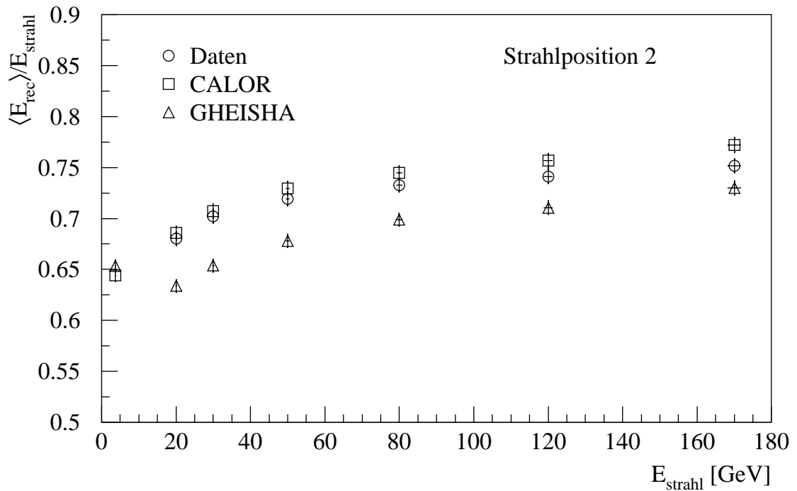
Abbildung 6.8: Verhältnis aus mittlerer rekonstruierter Energie und Strahlenergie \langle E_{rec} \rangle / E_{strahl} für Pionen in Strahlposition 1 und 2.
