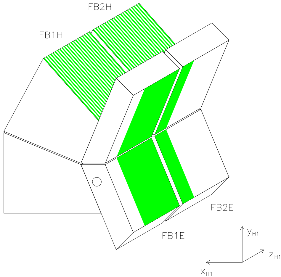
Abbildung 4.9: Perspektivische Ansicht des Testkalorimeters. Ein Loch in der vorderen Stahlplatte des unteren FB1E-Moduls erlaubt den direkten Einschuss ins FB1H-Kalorimeter.
