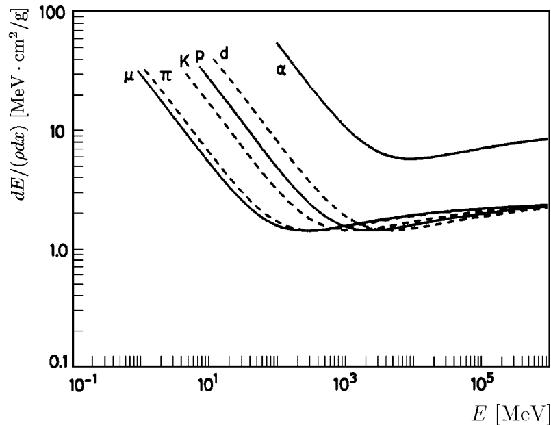
Abbildung 2.5: Ionisationsverlust schwerer Teilchen als Funktion der Energie [Leo87]
