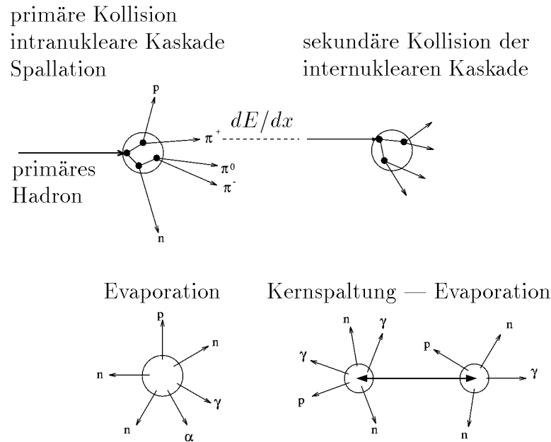
Abbildung 2.6: Schema einer Hadron-Kern-Wechselwirkung mit nachfolgender Evaporation bzw. Kernspaltung, in Anlehnung an eine Abbildung in [Brü87]
