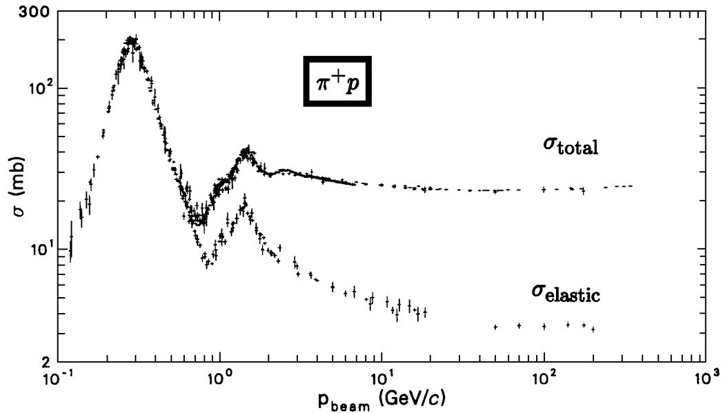
Abbildung 2.4: Wirkungsquerschnitt für Pion-Proton-Streuung [Par90]
