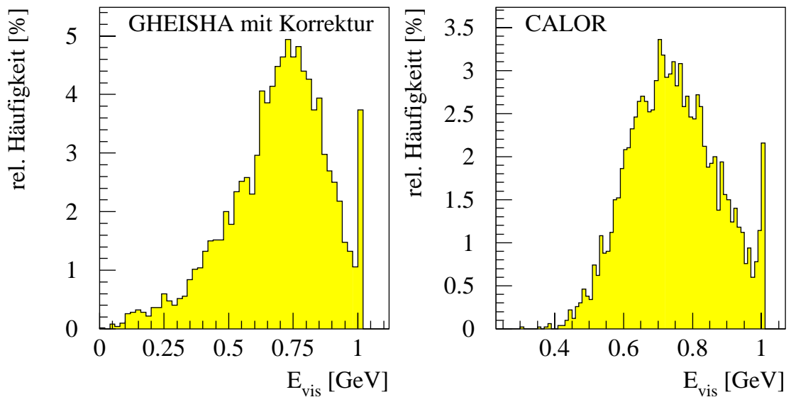
Abbildung A.2: Verteilung der nachweisbaren Energie E_{vis} bei durch 1 GeV Protonen ausgelösten Schauern in einem Eisenblock, Simulation mit korrigiertem GHEISHA und CALOR.
