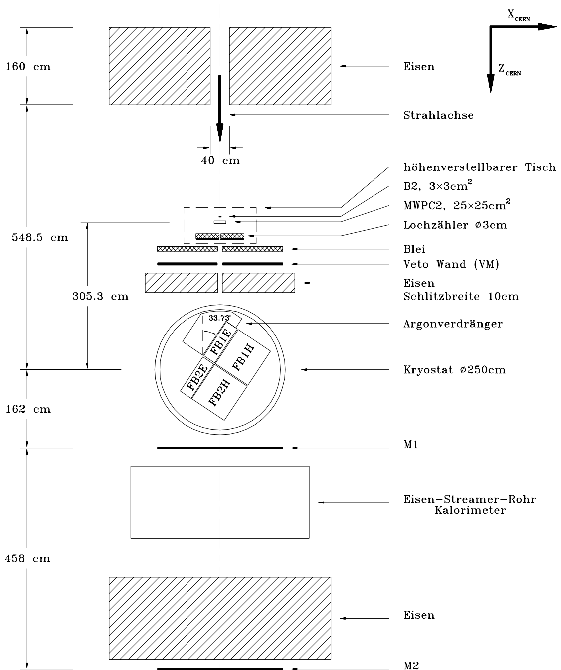
Abbildung 4.8: Aufbau des Kalorimeterteststands am H6-Teststrahl des CERN SPS.
