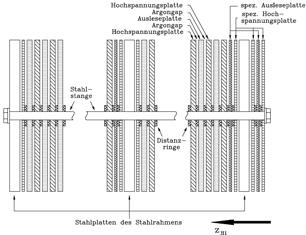
Abbildung 4.3: Schnitt durch ein FBE-Modul des H1-Detektors parallel zur Strahlachse
