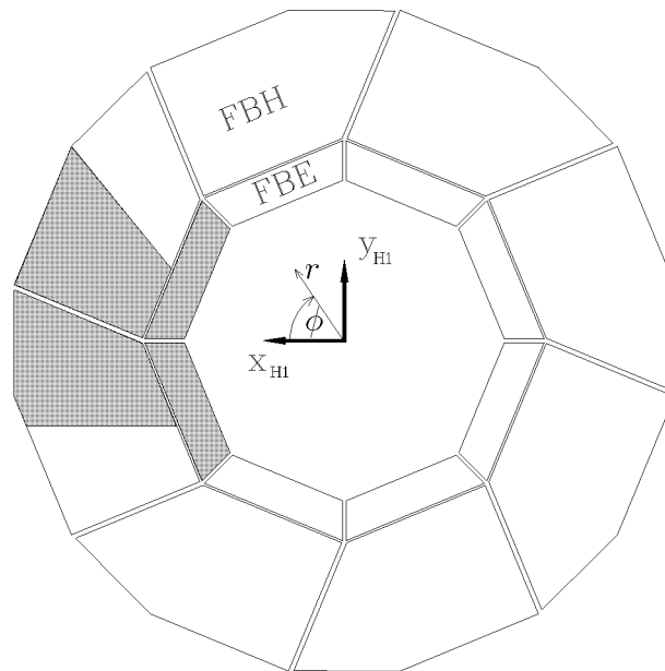
Abbildung 4.2: Schnitt durch das Kalorimeter des H1-Detektors senkrecht zur Strahlachse, der schraffierte Bereich markiert den Teil, der als Testkalorimeter am CERN verwendet wurde.
