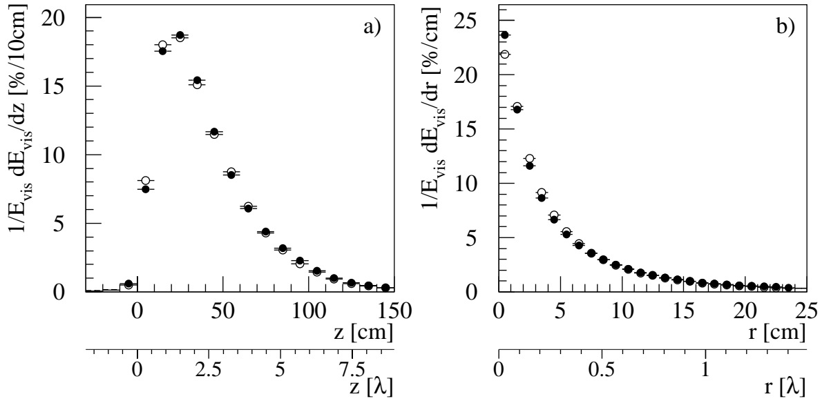
Abbildung 3.3: a) longitudinale und b) transversale Verteilung der Energiedeposition von hadronischen Schauern in Eisen, ausgelöst durch 20 GeV Pionen, offene Symbole GHEISHA, volle Symbole CALOR, \lambda = nukleare Absorptionslänge
