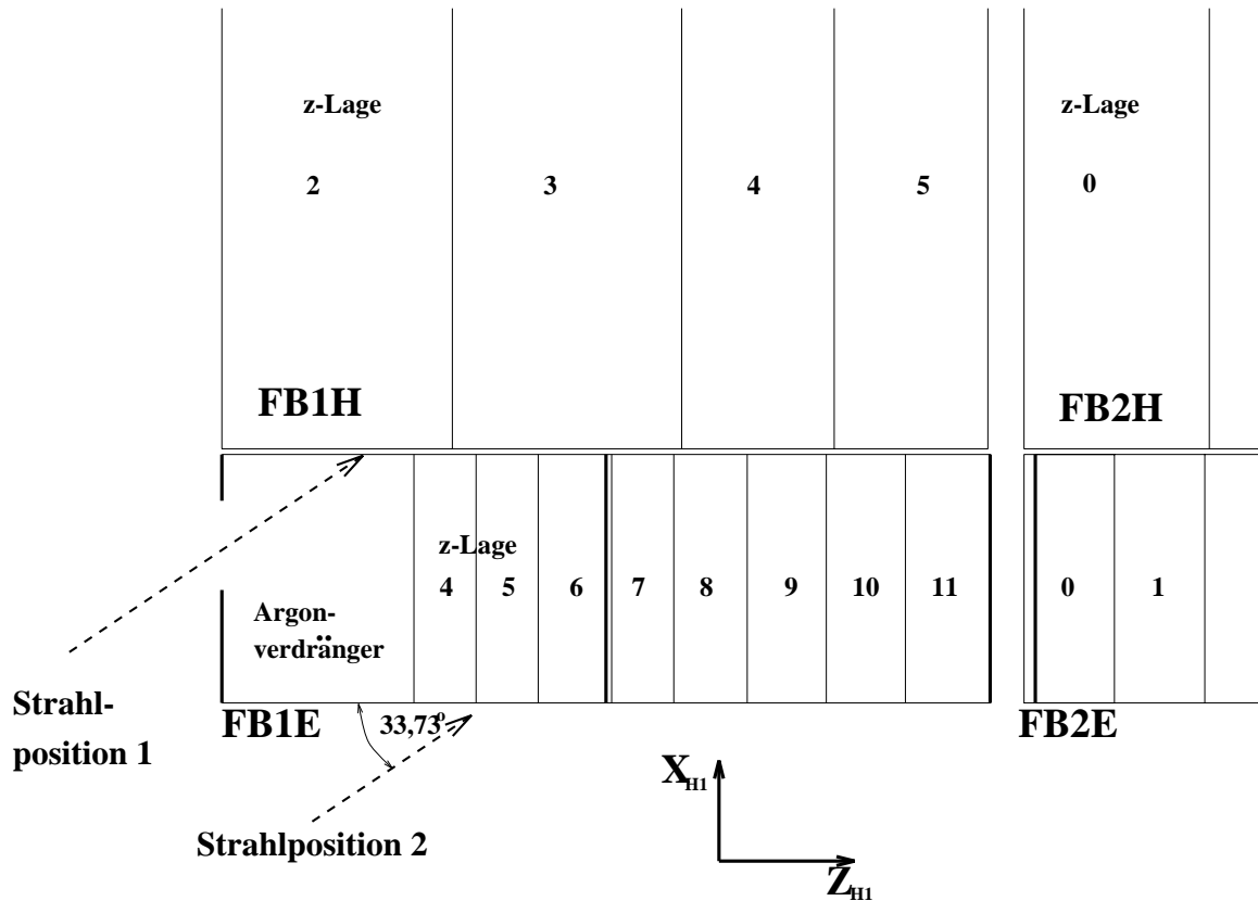
Abbildung 4.10: Schnitt durch das Testkalorimeter auf der Höhe des Lochs in der Frontplatte des unteren FB1E-Moduls, Strahlpositionen und Numerierung der z-Lagen.
