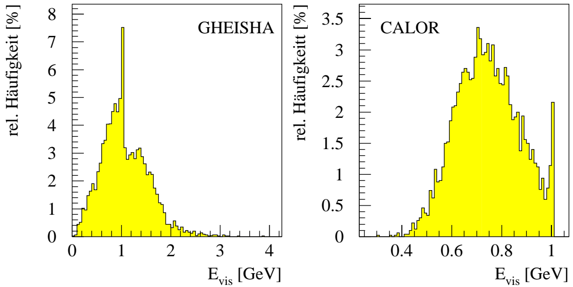
Abbildung A.1: Verteilung der nachweisbaren Energie E_{vis} bei durch 1 GeV Protonen ausgelösten Schauern in einem Eisenblock, Simulation mit GHEISHA und CALOR.
