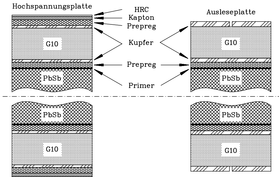
Abbildung 4.4: Schichtfolge der Materialien in den Absorberplatten des FBE Kalorimeters.
