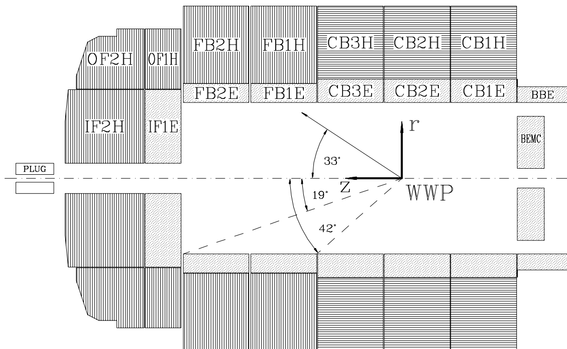
Abbildung 4.1: Schnitt durch das Kalorimeter des H1-Detektors parallel zur Strahlachse.
