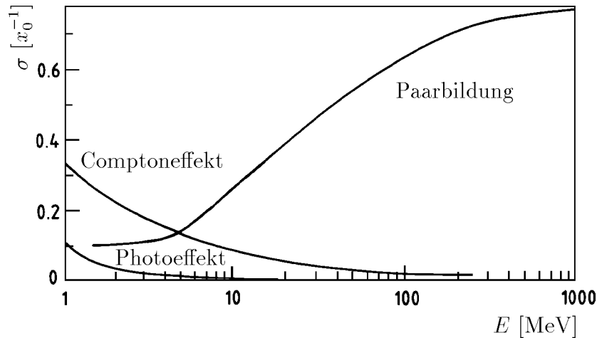
Abbildung 2.2: Wirkungsquerschnitt \sigma der Photonabsorption in Blei als Funktion der Photonenergie, gemessen in inversen Strahlungslängen x_0^{-1} [Par90].
