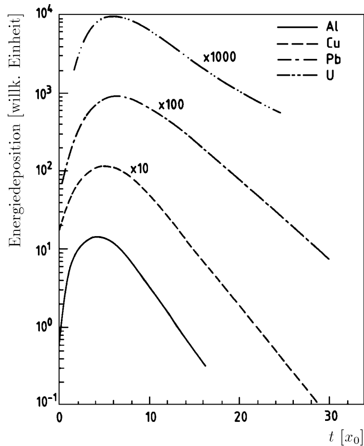
Abbildung 2.3: Longitudinales Schauerprofil für 6 GeV Elektronen in Aluminium, Kupfer, Blei und Uran [Fab85].
