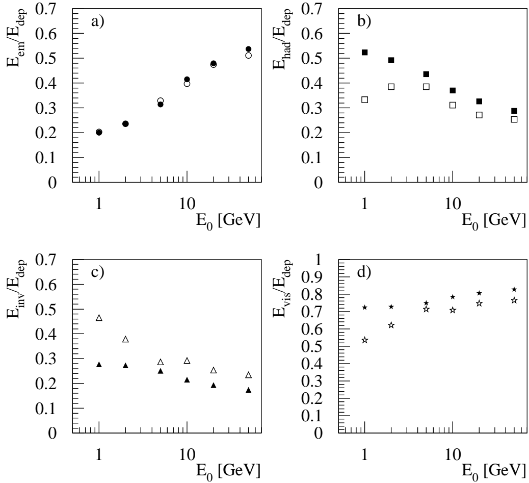
Abbildung 3.1: Vergleich der relativen Anteile der in Abschnitt 2.2.2 erläuterten Schauerkomponenten an der gesamten deponierten Energie für Pionen in Abhängigkeit von der Primärenergie für GHEISHA und CALOR, offene Symbole GHEISHA, volle Symbole CALOR, a) elektromagnetischer Anteil E_{em}/E_{dep} , b) hadronischer Anteil E_{had}/E_{dep} , c) nicht nachweisbarer Anteil E_{inv}/E_{dep} , d) nachweisbarer Anteil E_{vis}/E_{dep} = (E_{em} + E_{had})/E_{dep} . Die statistischen Fehler sind kleiner als die Symbole.
