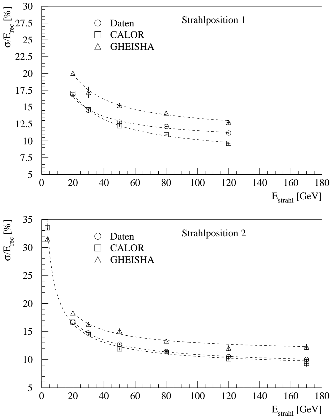
Abbildung 6.10: Relative Auflösung bei der Energiemessung von hadronischen Schauern für Daten [Kor94] und Simulationen mit GHEISHA bzw. CALOR. Die Kurven zeigen Anpassungen an die erhaltenen Werte, siehe Text.
