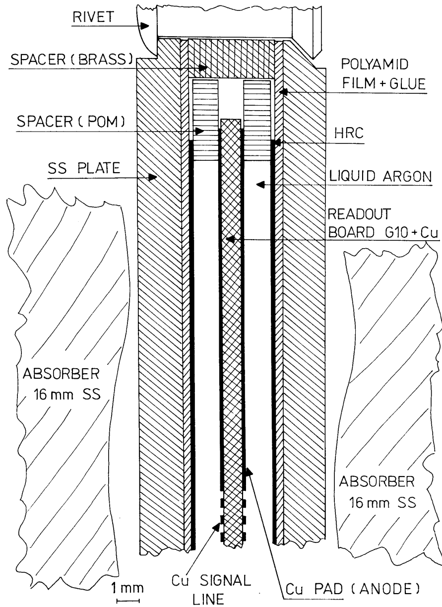
Abbildung 4.7: Schnitt durch eine Auslezelle des FBH-Kalorimeters.
