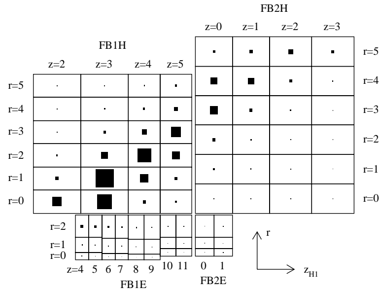
Abbildung 6.1: Verteilung der mittleren Energiedeposition in der r - z_{H1} -Ebene in hadronischen Schauern von 20 GeV Pionen bei Strahlposition 1, Simulation mit CALOR.
