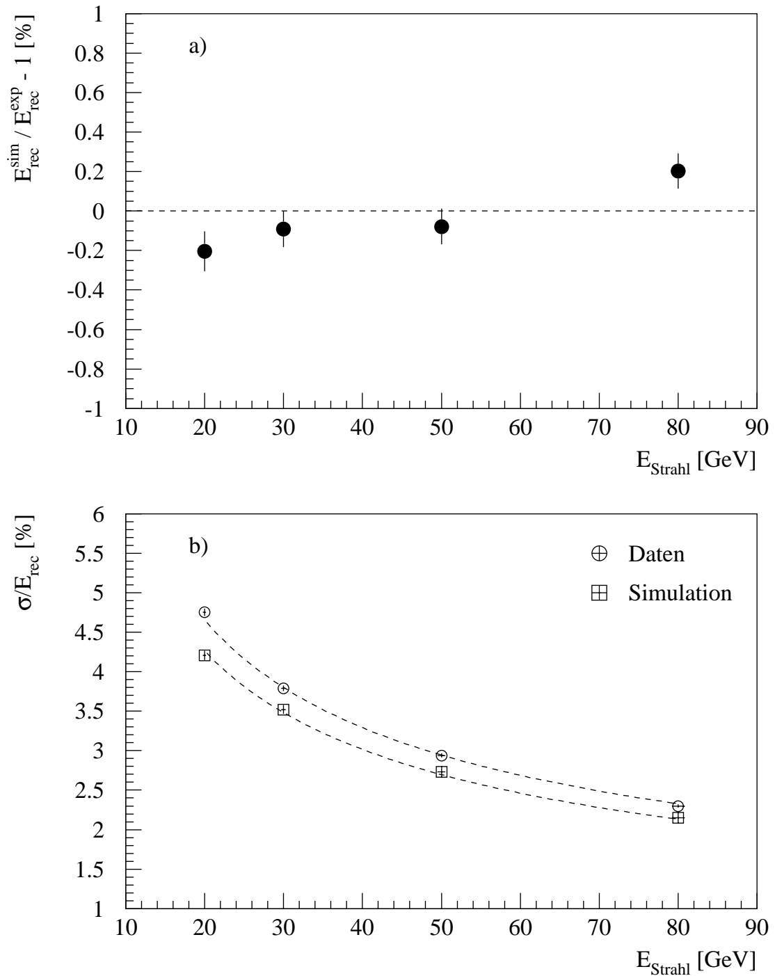
Abbildung 5.7: Vergleich zwischen den Resultaten der Kalibrationsmessungen mit Elektronen [Kor94] und denen der Simulation, a) Verhältnis der rekonstruierten Energien, b) Vergleich der relativen Auflösungen
