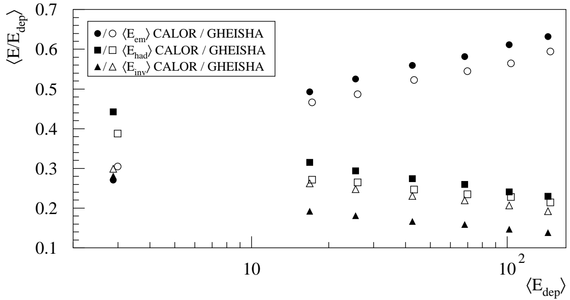
Abbildung 6.12: Mittlere Anteile der verschiedenen in Abschnitt 2.2.2 diskutierten Schauerkomponenten an der gesamten deponierten Energie E_{dep} in Abhängigkeit von E_{dep} für Simulationen mit CALOR und GHEISHA bei Strahlposition 2.
