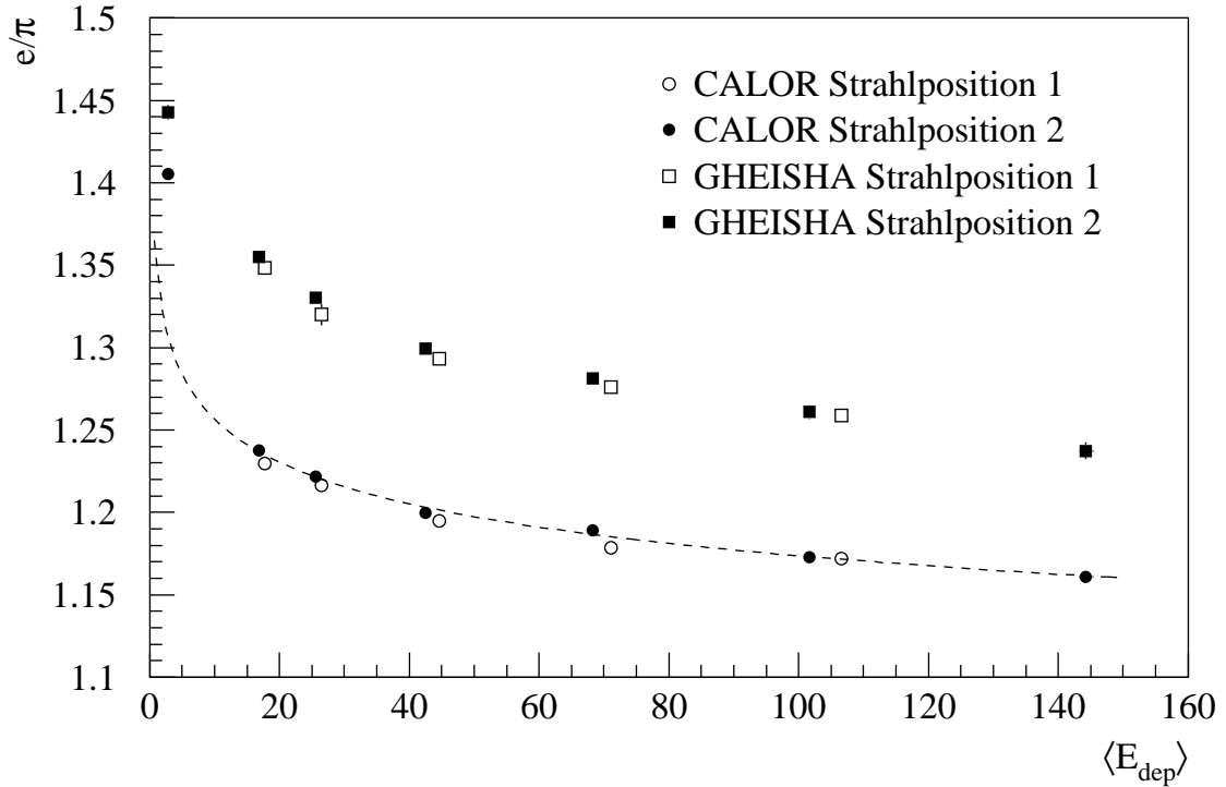
Abbildung 6.11: Verhältnis e/\pi in Abhängigkeit von der mittleren im Kalorimeter deponierten Energie \langle E_{dep} \rangle simuliert mit CALOR und GHEISHA für die Strahlpositionen 1 und 2. Die Kurve zeigt eine Anpassung gemäß Gleichung 2.7.
