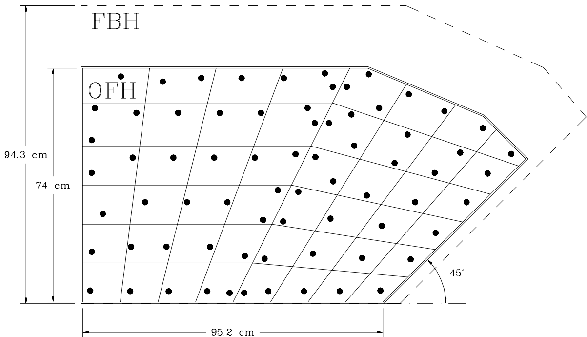
Abbildung 4.6: Skizze einer OFH- bzw. FBH-Auslesekarte, Einteilung der OFH-Auslesekarte in Pads, die schwarzen Kreise stellen die Nieten der OFH-Auslesekarte dar.
