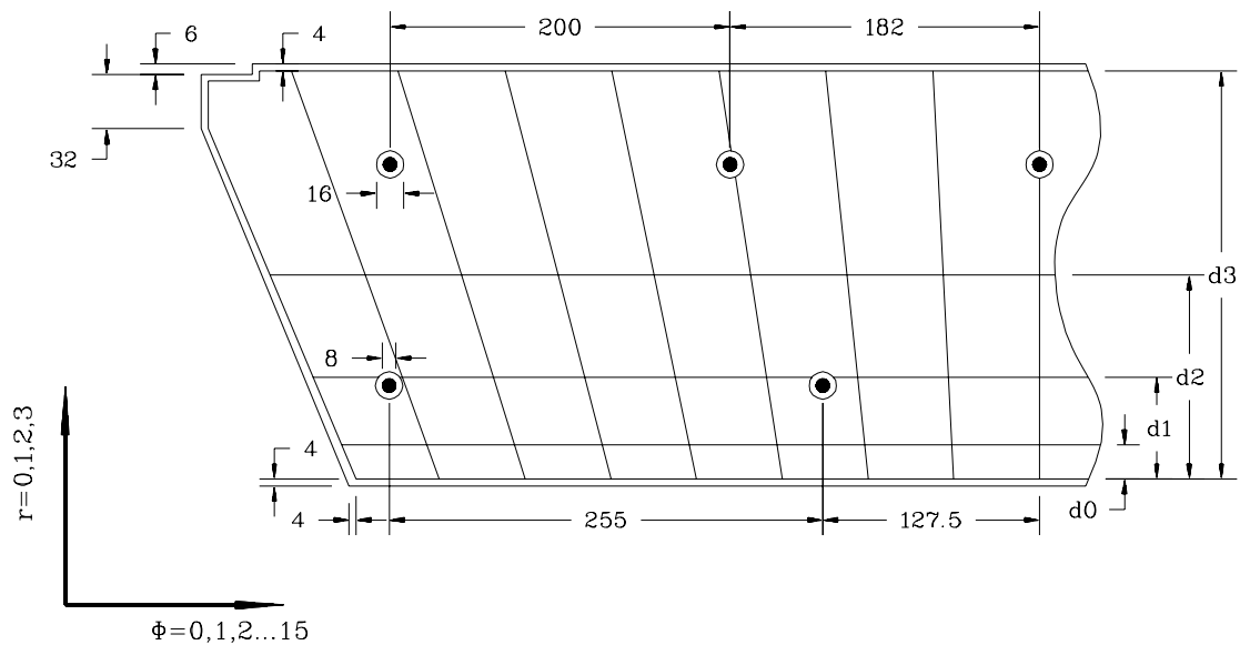
Abbildung 4.5: Aufteilung einer Ausleseplatte des FB2E-Kalorimeters in unabhängige Auslesezellen, alle Maße in mm, die schwarzen Punkte zeigen die Bohrungen für die Stahlstangen. d_0 - d_3 : siehe Tabelle 4.2
